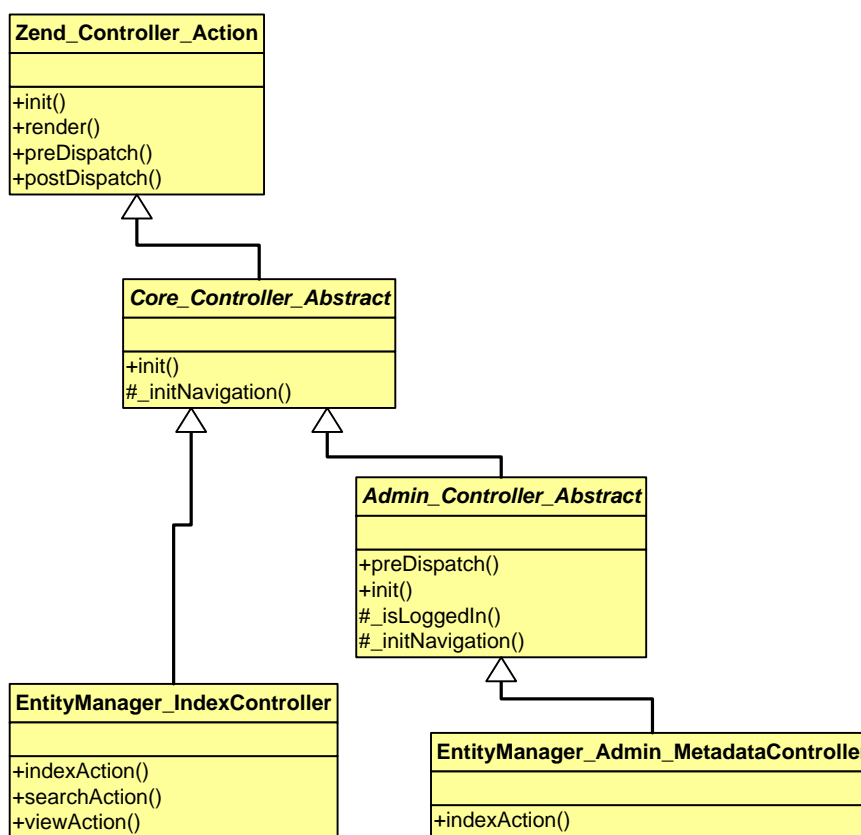
Obrázek 8.2: Abstraktní třídy kontrolerů
