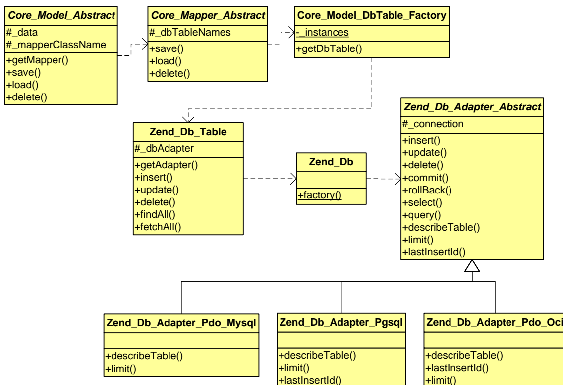
Obrázek 8.5: Využití Zend_Db_Adapter pro přístup k rozhraní databáze
