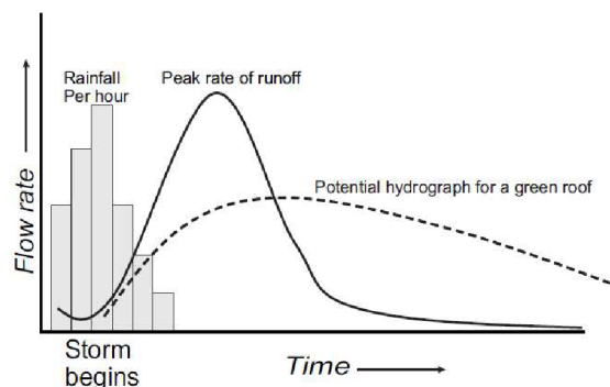
Obr. 44: Křivka odtoku srážek běžná vs. vegetační střeška [30]
