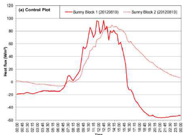
Obr. 31: Tepelný tok klasickou střechou 1 – nezateplená 2 – zateplená [24]
