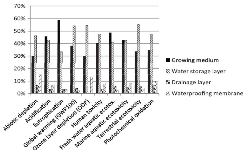
Obr. 22: Podíl funkčních vrstev střechy na celkové emisí [22]
