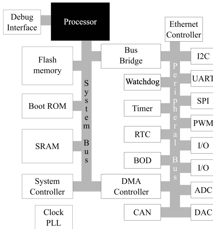
Obrázek 3.1: Schéma mikrokontroleru [30]
