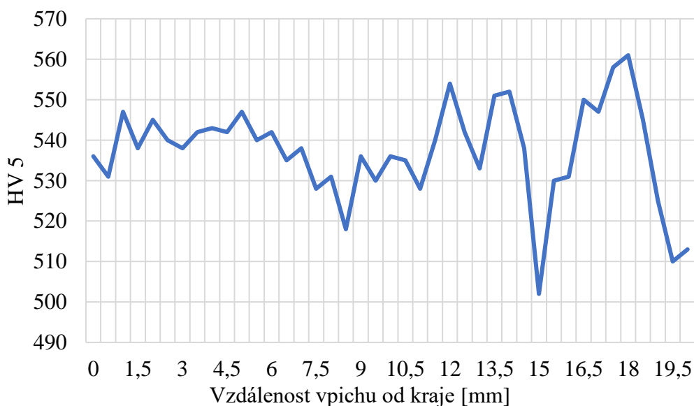
Obr. 46 graf průběhu tvrdosti vzorku 2.
