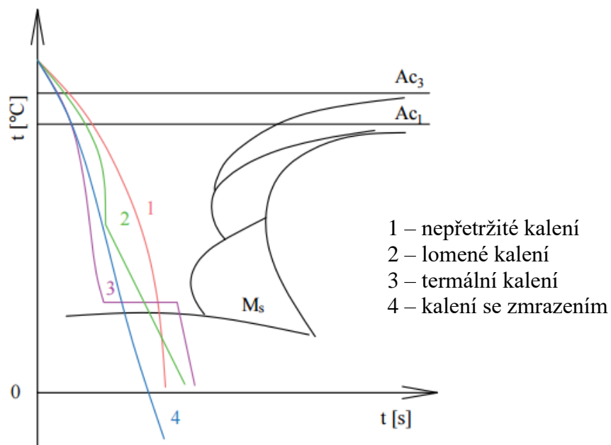
Obr. 24 Druhy kalení. [15]
