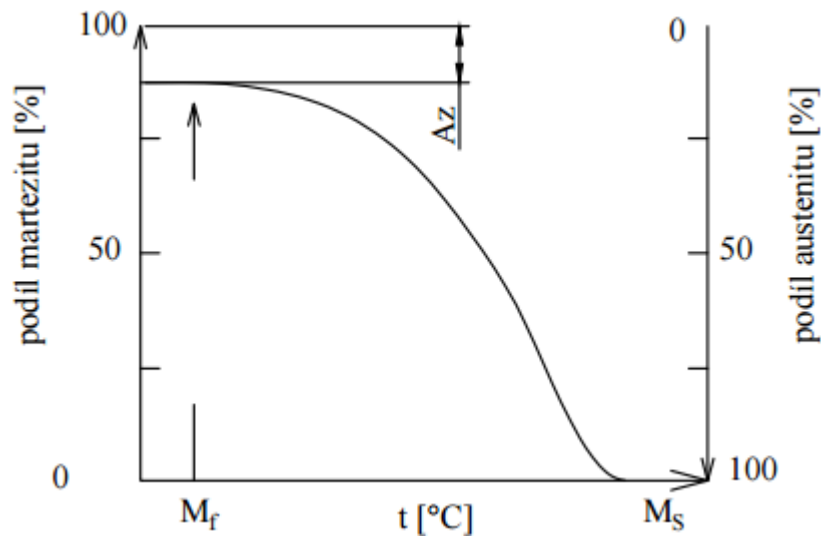
Obr. 20 Schéma martenzitické křivky oceli. [13]
