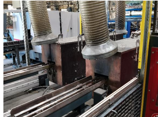
Obr. 5 indukční přehřev přířezů.
