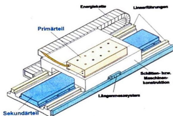
Obr. 2.5: Lineárny motor [2]
