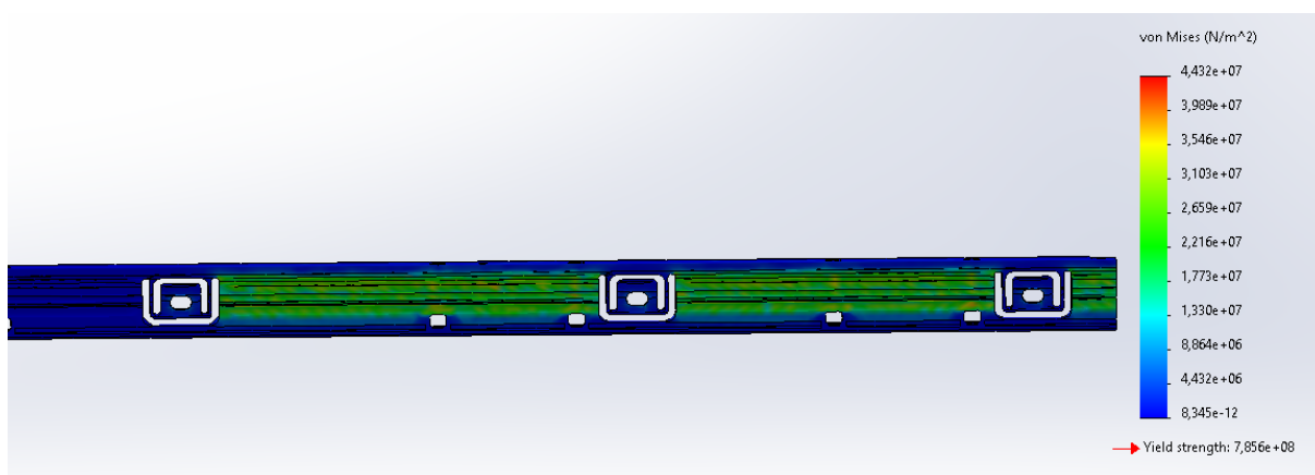
Obr. 5.15: Napätie v dilatačnej podložke z ocele 18NiCr5-4
