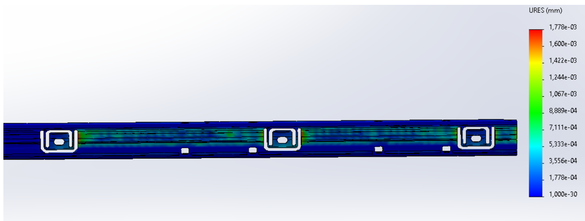
Obr. 5.13: Deformácia v dilatačnej podložke z duralu
