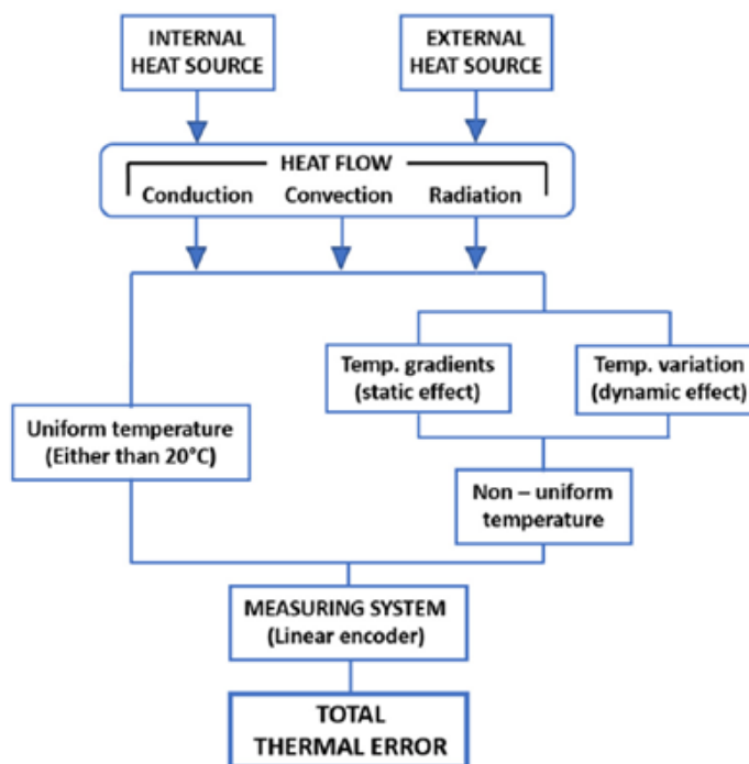
Obr. 4.1: Termálne účinky v integrovaných meracích systémoch [10]
