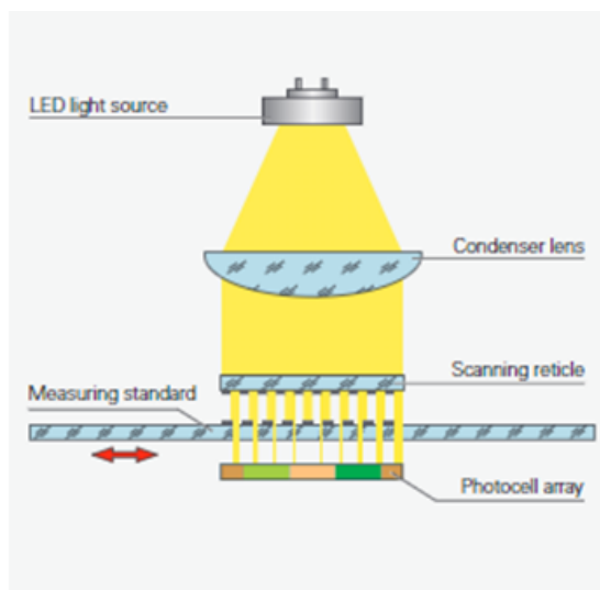
Obr. 3.5: Princíp zobrazovacieho snímania [3]
