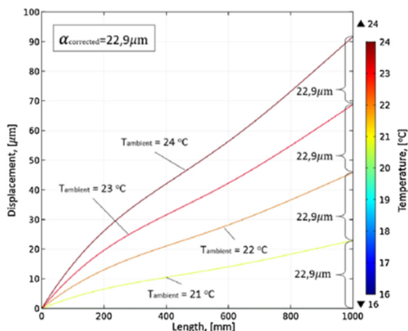
Obr. 4.4: Celkový posun pozdĺž ocelej stupnice pri rôznych jednotných teplotách okolia [10]
