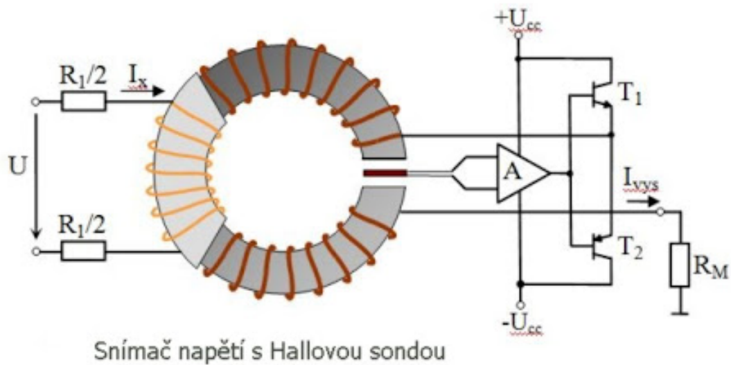
Obr. 1.9: Snímač napätia s Hallovou sondou [8]
