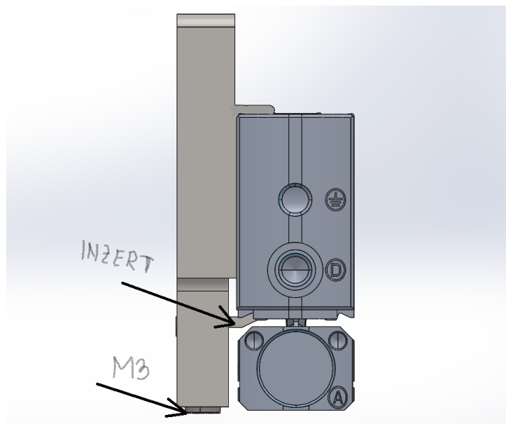
Obr. 5.7: Konštrukčný variant č. 3: skrutka M3 pre utiahnutie inzertu.
