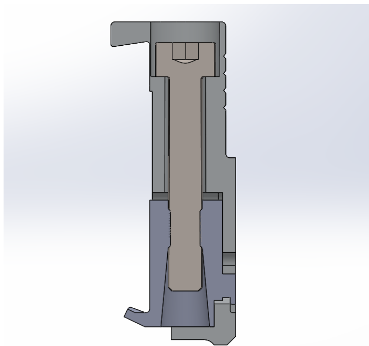
Obr. 5.11: Spojenie inzertu a podložky
