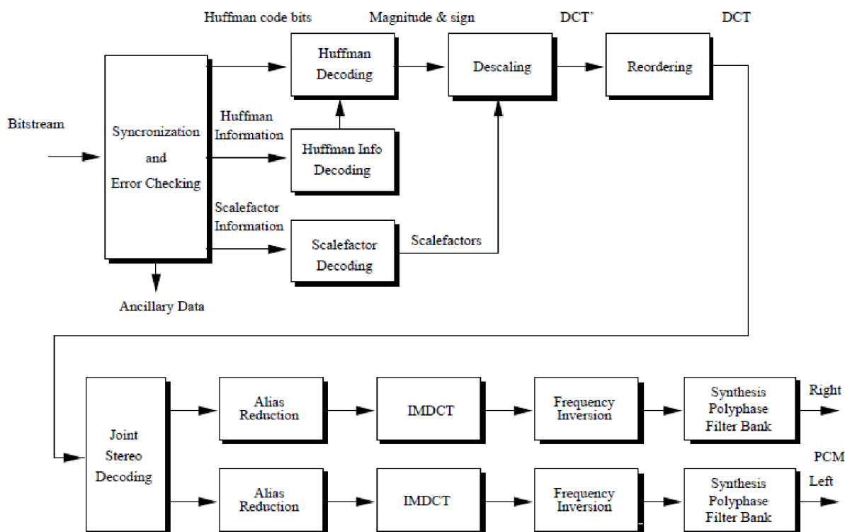
Obrázek 5: Části dekodéru [3]
