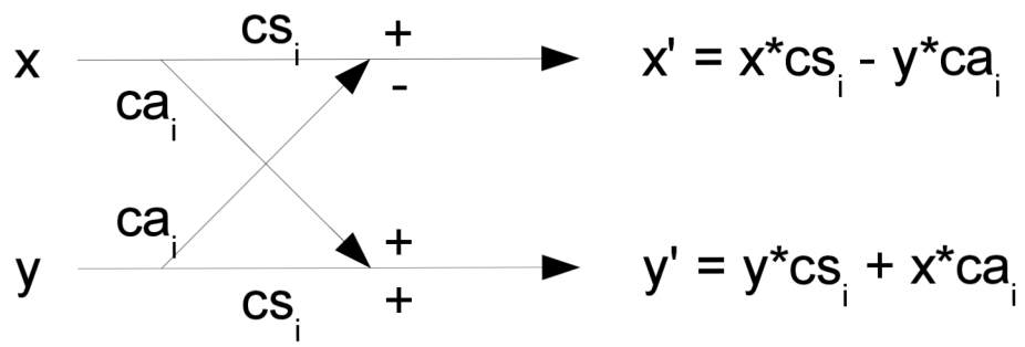
Obrázek 14: Motýlková transformace
