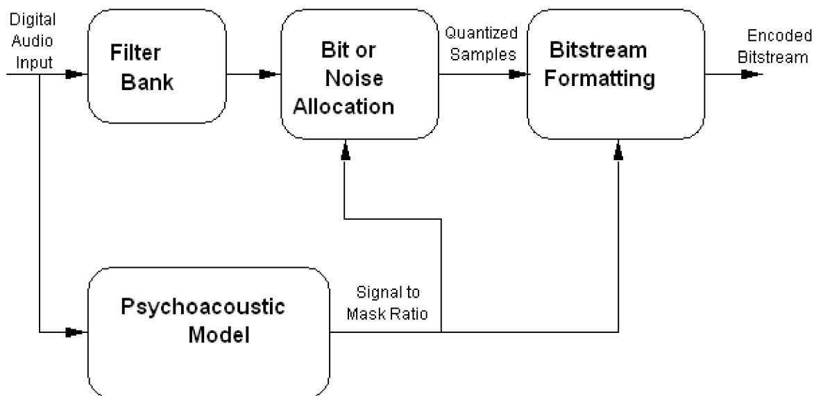
Obrázek 4: Struktura enkodéru [1]
