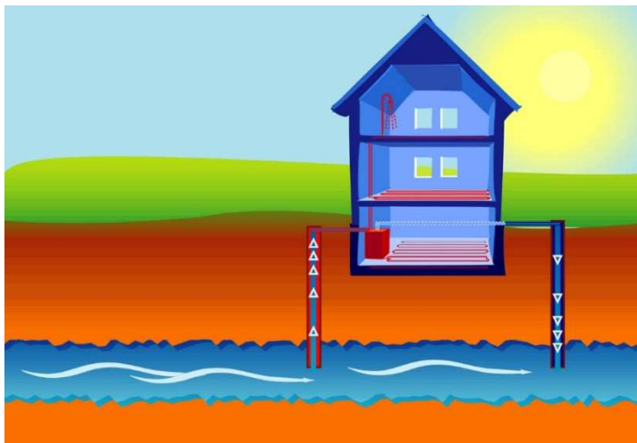
Obr. 15: Schéma: tepelné čerpadlo – voda/voda [22]
