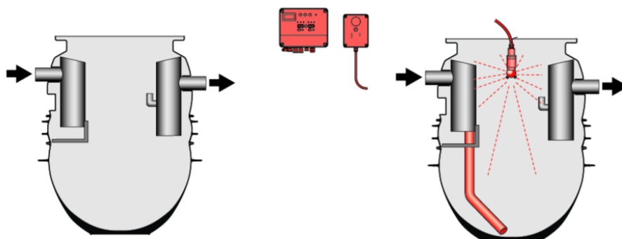
Obrázek 14: Základní a složitější provedení tukového odlučovače z polyetylemu (ACO, ©2023)
