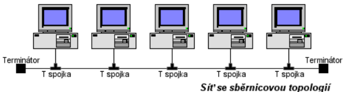
Obrázek 2-4: Síť se sběrniceovou topologií
