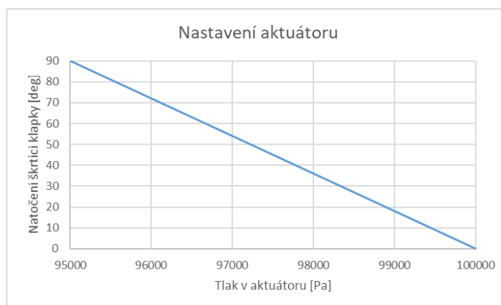
Graf 4-8 Nastavení závislosti měřeného tlaku na natočení škrtkové klapky v aktuátoru
