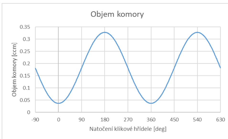
Graf 4-3 - Objem komory v závislosti na natočení klikového hřídele
