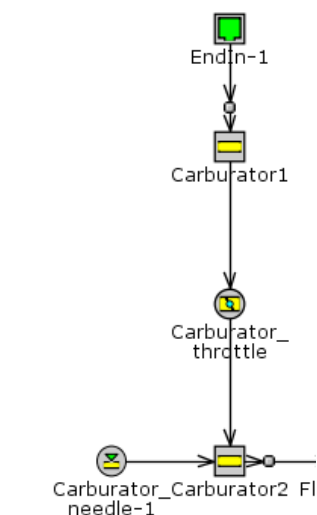
Graf 4-5 Model karburátoru motoru Aixro XR 50
