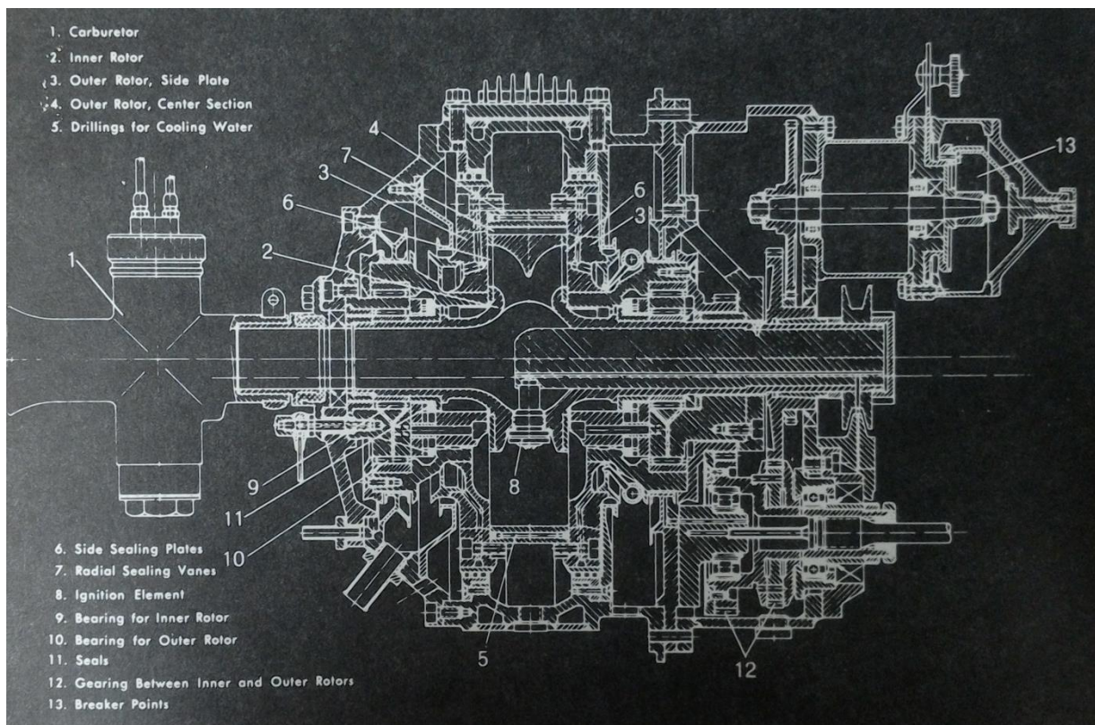
Obr. 1-3 Řez motorem DKM 54, 1 - Karburátor, 2 - Vnitřní rotor, 3 - Vnější rotor boční strany, 4 - Vnější rotor střední část, 5 - Vodní kanál, 6 - Boční těsnící desky, 7 - Radiální těsnění vnitřního rotoru, 8 - Zapalovací svíčka, 9 - Ložisko vnitřního rotoru, 10 - Ložisko vnitřního rotoru, 11 - radiální těsnění hřídele, 12 - ozubené soukolí převodu vnějšího a vnitřního rotoru s poměrem 3:2, 13 - Magneto-elektrické zapalování
