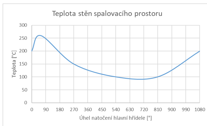
Graf 4-12 Závislost teploty stěn spalovacího prostoru na natočení hlavní hřídele – nulový bod značí horní úvrat' expanze.
