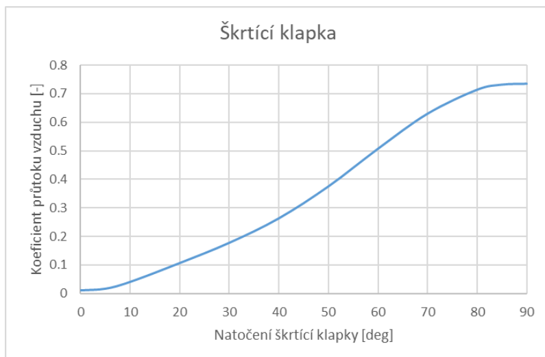
Graf 4-4 Závislost koeficientu průtoku vzduchu na natočení škrťací klapky
