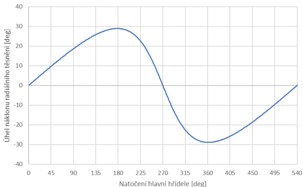
Obr. 11 Úhel náklonu radiálního těsnění pro K=6,2 - návrhový motor
