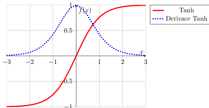
Obr. 1.5: Průběh Hyperbolické tangenty a její derivace
