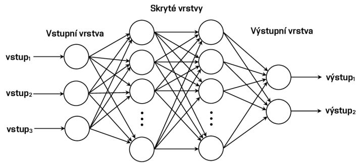
Obr. 1.1: Struktura umělé neuronové sítě s 2 skrytými vrstvami
