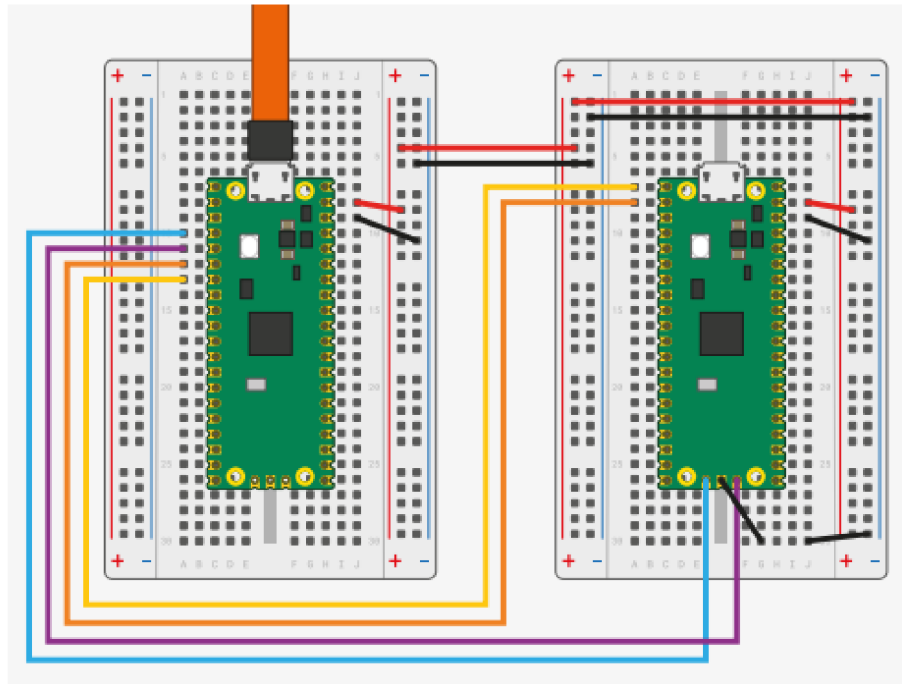
Obr. A.3: Propojení dvou Raspberry pro ladění SW [3]
