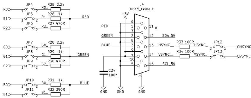
Obr. A.6: Zapojení obrazového VGA výstupu [1]
