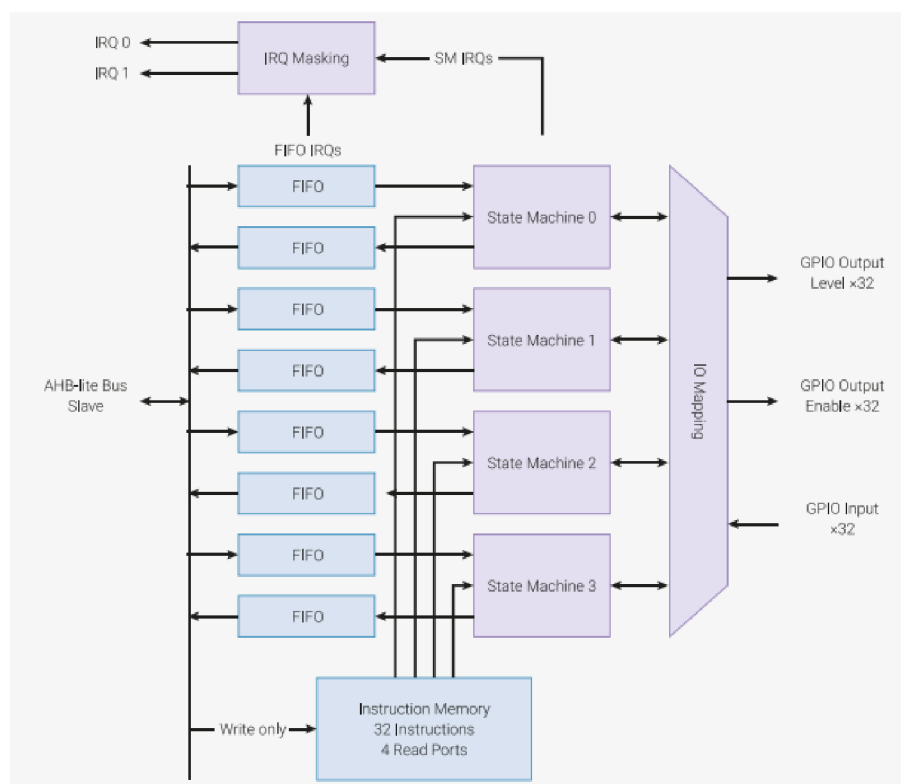
Obr. A.2: Diagram PIO bloku [4]
