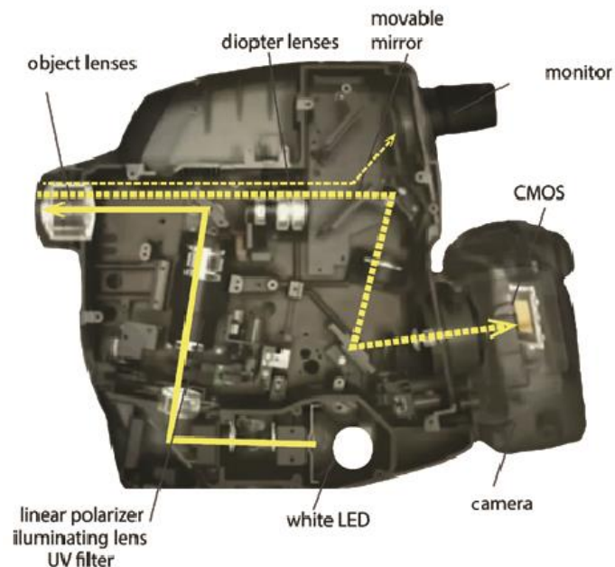
Obr. 2 - 18 schéma optických dráh v hlave kamery [26]
