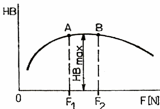
Obr. 2.2 závislost tvrdosti podle Brinella na zatěžující síle [8]
