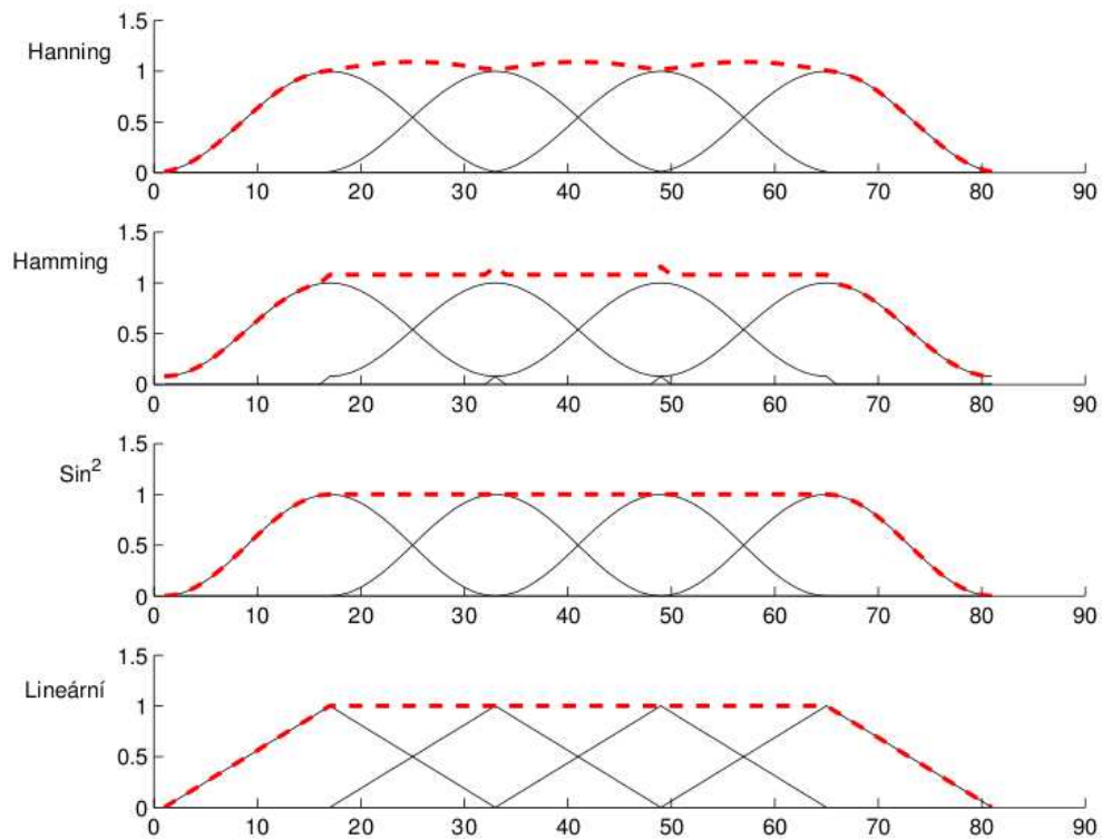
Obrázek 4.3: Okénkovací funkce
