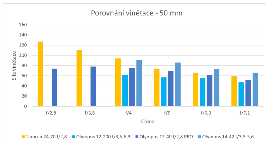
Obr. 4.3.1-14 Graf porovnání vinětace 50 mm.
