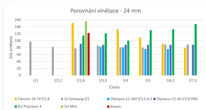
Obr. 4.3.1-10 Graf porovnání vinětace 24 mm.
