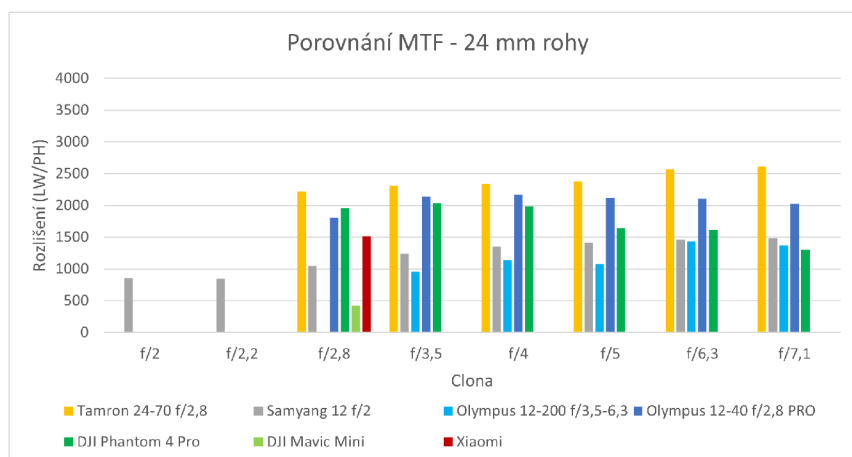
Obr. 4.3.3-17 Graf porovnání MTF 24 mm rohy.
