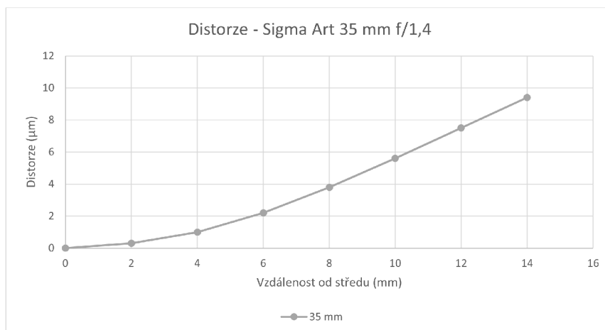
Obr. 4.3.4-2 Graf distorze objektiv Sigma Art 35 mm f/1,4.
