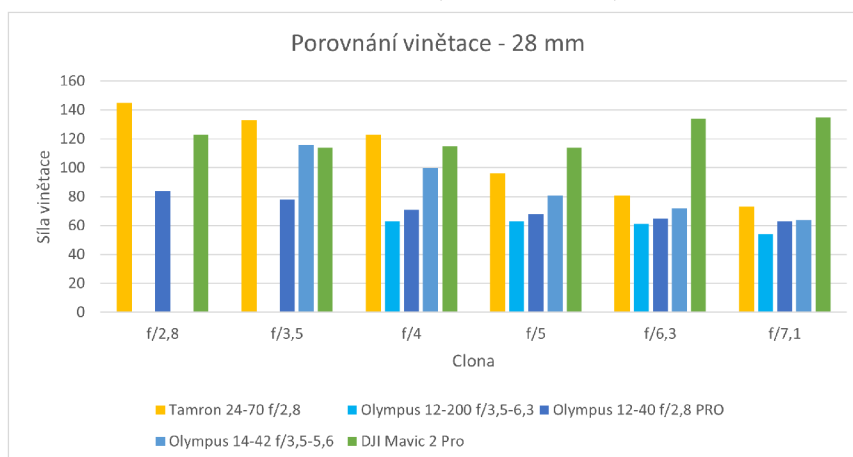
Obr. 4.3.1-11 Graf porovnání vinětace 28 mm.
