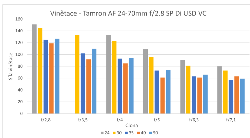
Obr. 4.3.1-1 Graf vinětace objektiv Tamron 24-70 mm f/2.8.
