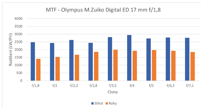
Obr. 4.3.3-11 Graf MTF objektiv Olympus 17 mm f/1,8.
