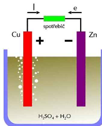
Obr. 6-2 Princip elektrochemického článku [14]
