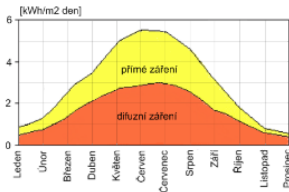
Obr. 3-3 Rozdíl mezi přímým a difúzním zářením [7]
