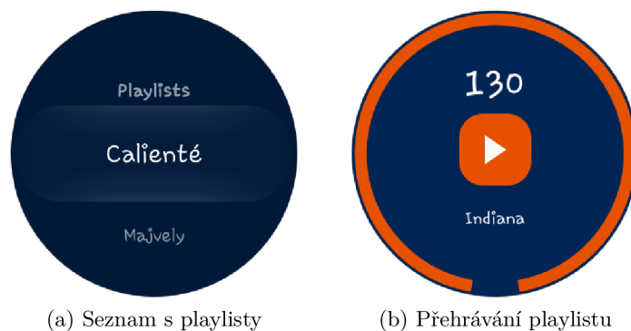
Obrázek 5.7: Aplikace MyMetronome
