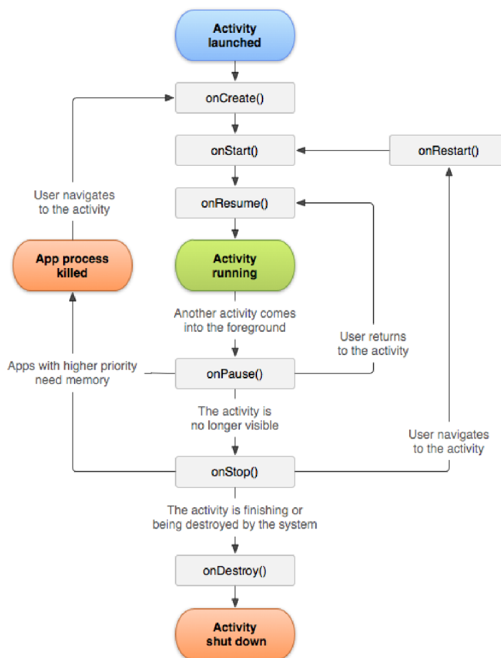
Obrázek 2.2: Životní cyklus aktivity. Převzato z [30].
