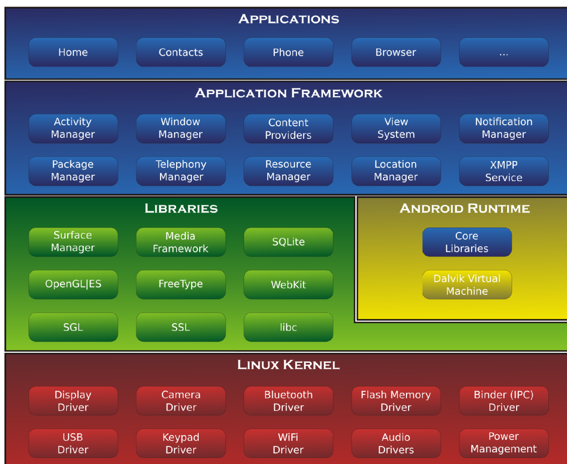
Obrázek 2.1: Architektura systému Android. Převzato z [19].
