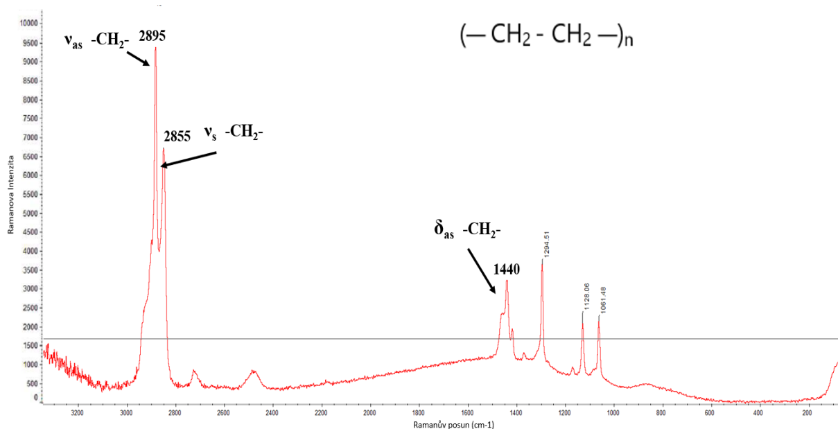
Obrázek 11: Změřené spektrum PE s označenými vibracemi; \nu_{as} – valenční asymetrická vibrace, \nu_s – valenční symetrická vibrace, \delta – rovinná deformační vibrace
