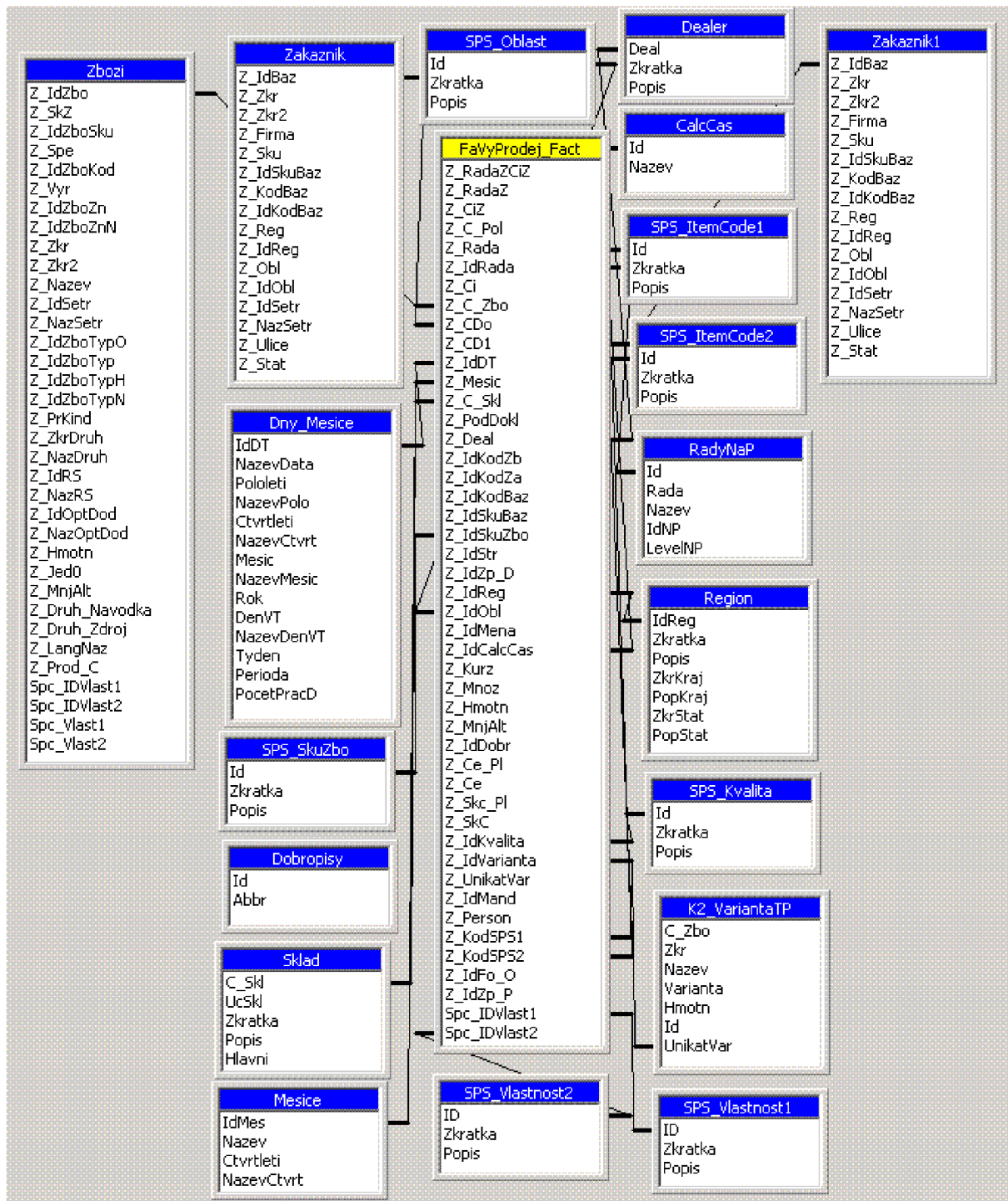
Obr. 5 Hvězdicové schéma datového trhu Prodej
