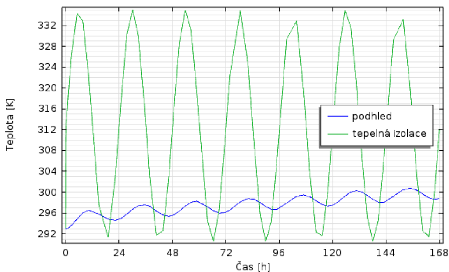
Obr. 27 Průběh povrchových teplot ve střešním plášti pasivní budovy, materiálové řešení s minerální vatou a sádkartonem v týdenním horizontu
