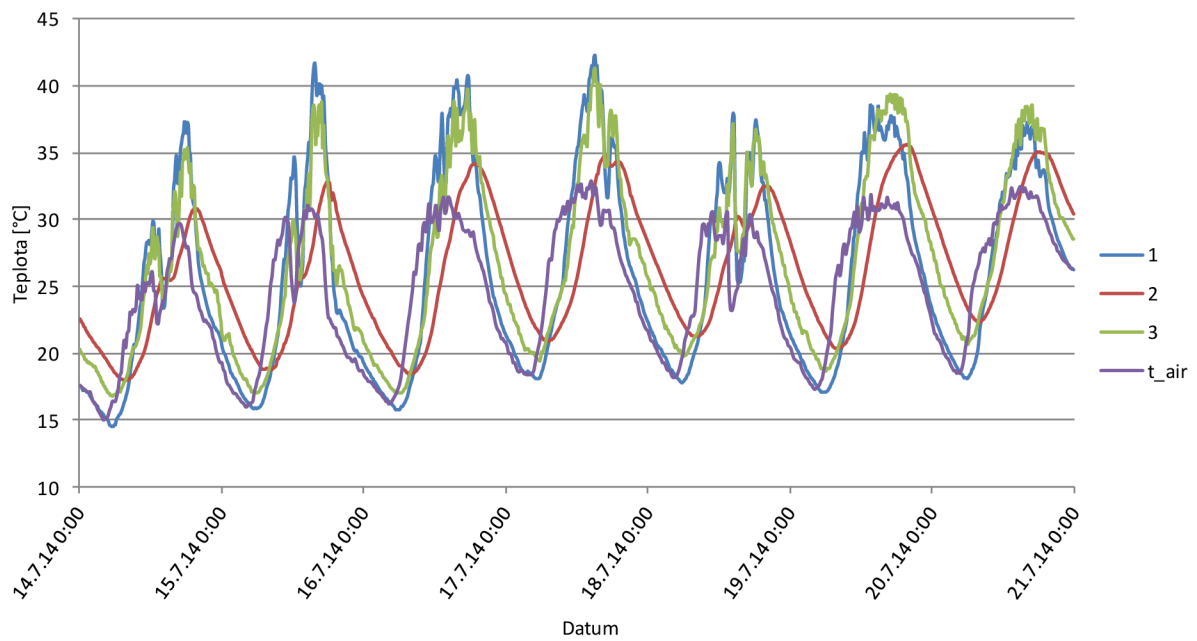
Obr. 43 Rozložení teplot v modelu střešního pláště – pole C (lisovaná sláma + šedá fólie)
