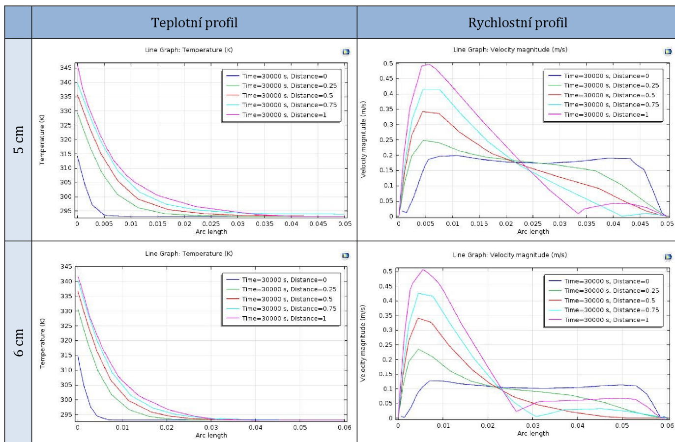
Obr. 56 Teplotní a rychlostní profily ve větrané dutině s velmi nízkou emisivitou povrchů (bez vlivu radiační složky); na svislé ose je vynesena teplota v Kelvinech, na vodorovné ose šířka dutiny, na levé straně je povrch horního pláště, na pravé straně je povrch spodního pláště
