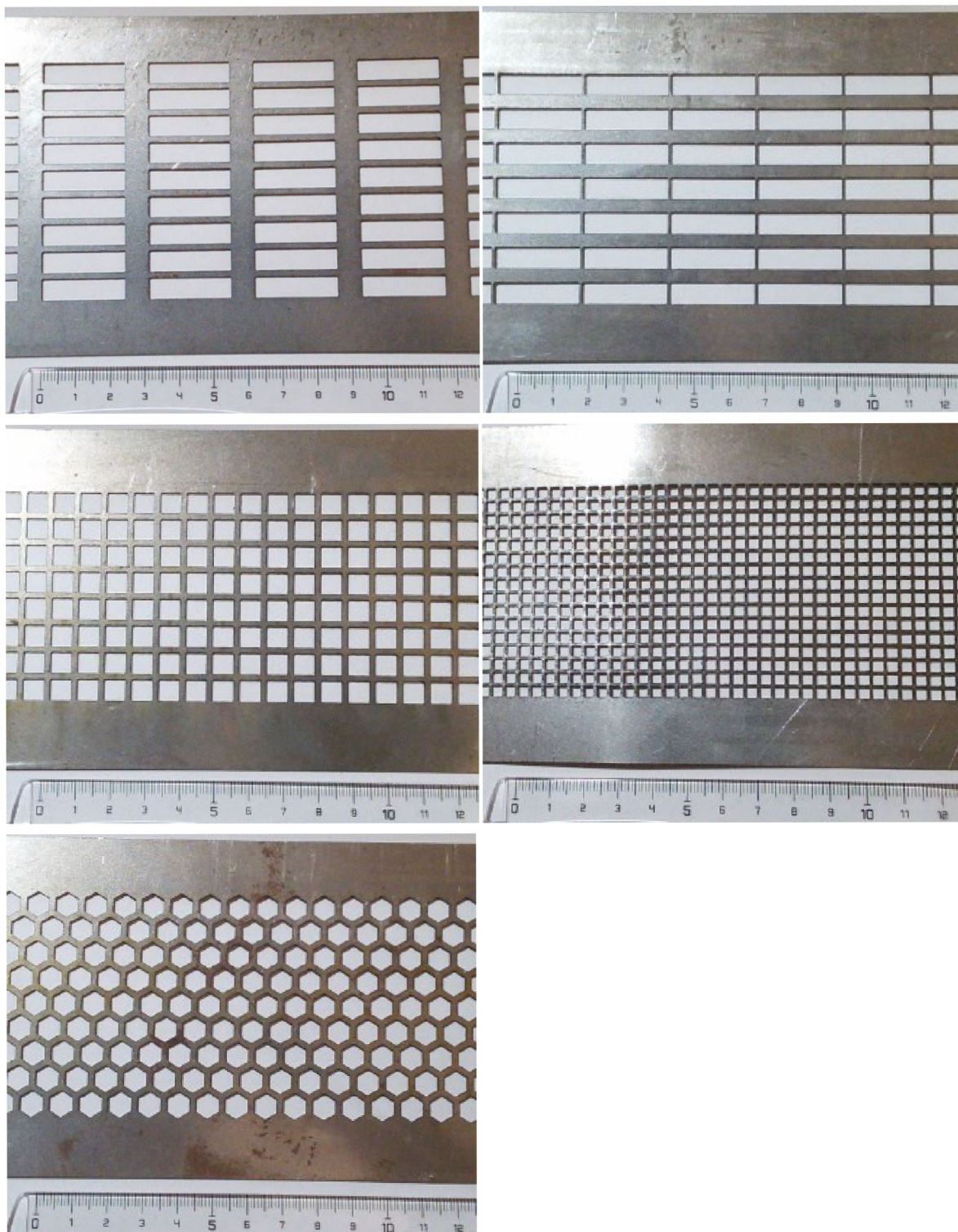
Obr. 71 Prototypy mřížek
