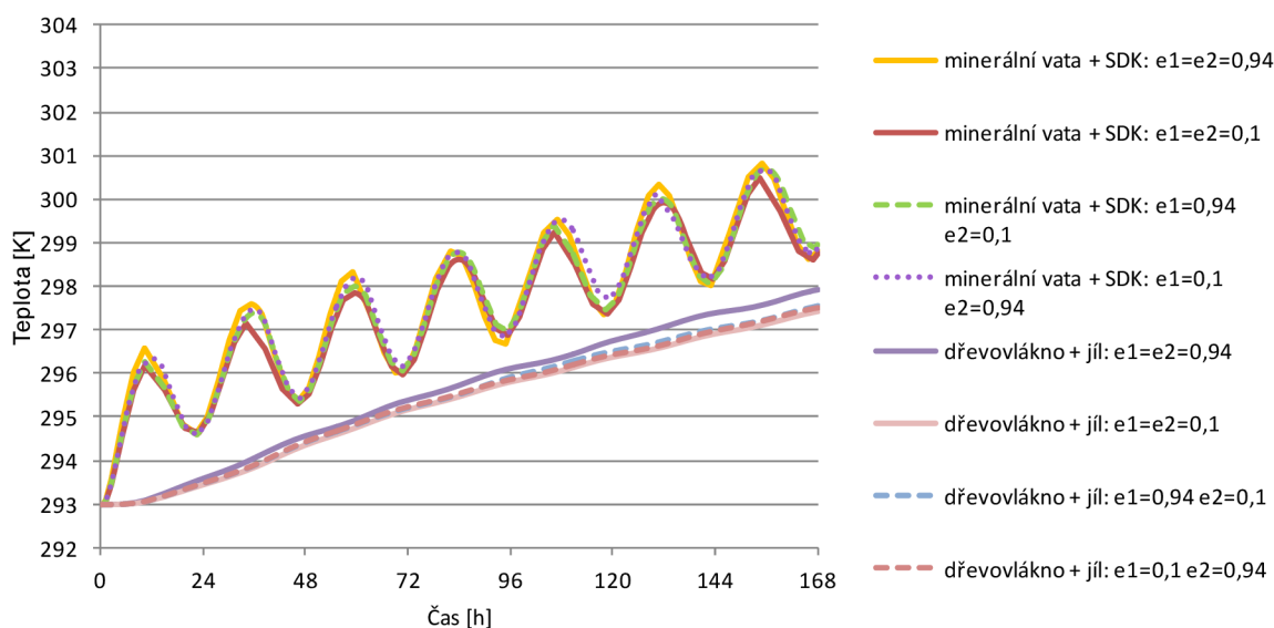
Obr. 35 Vliv reflexních povrchů: Teploty na lici stropního podhledu v periodě 7 dní
