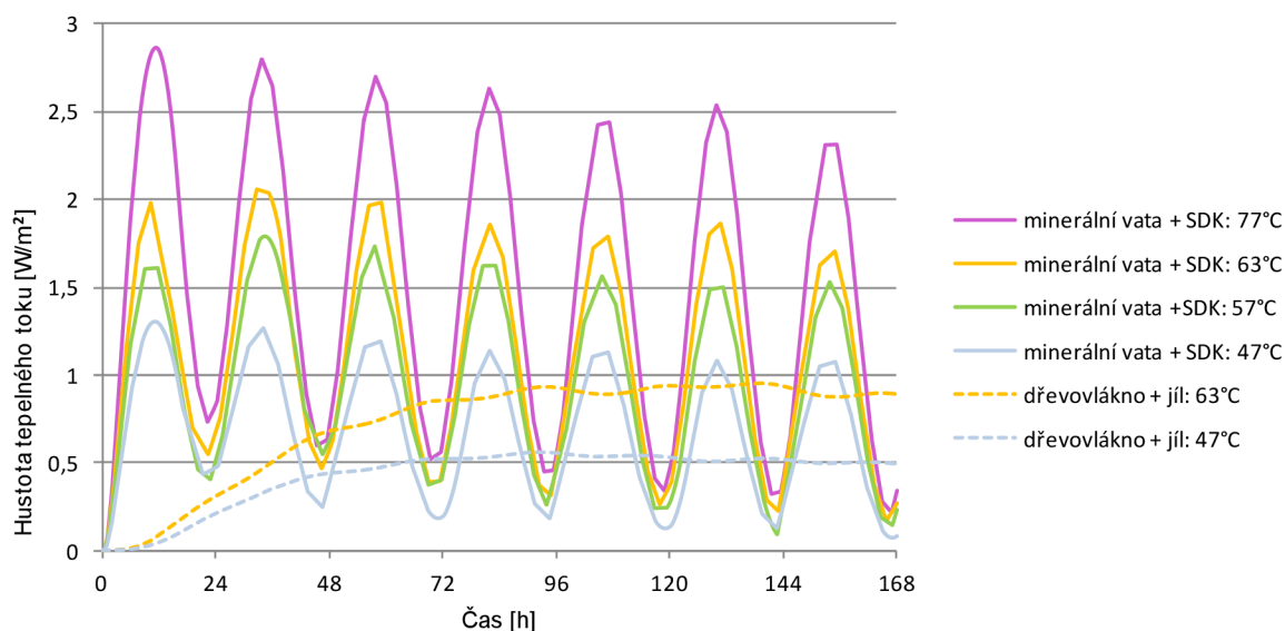
Obr. 39 Vliv barvy krytiny: Tepelné toky na líci stropního podhledu v periodě 7 dní
