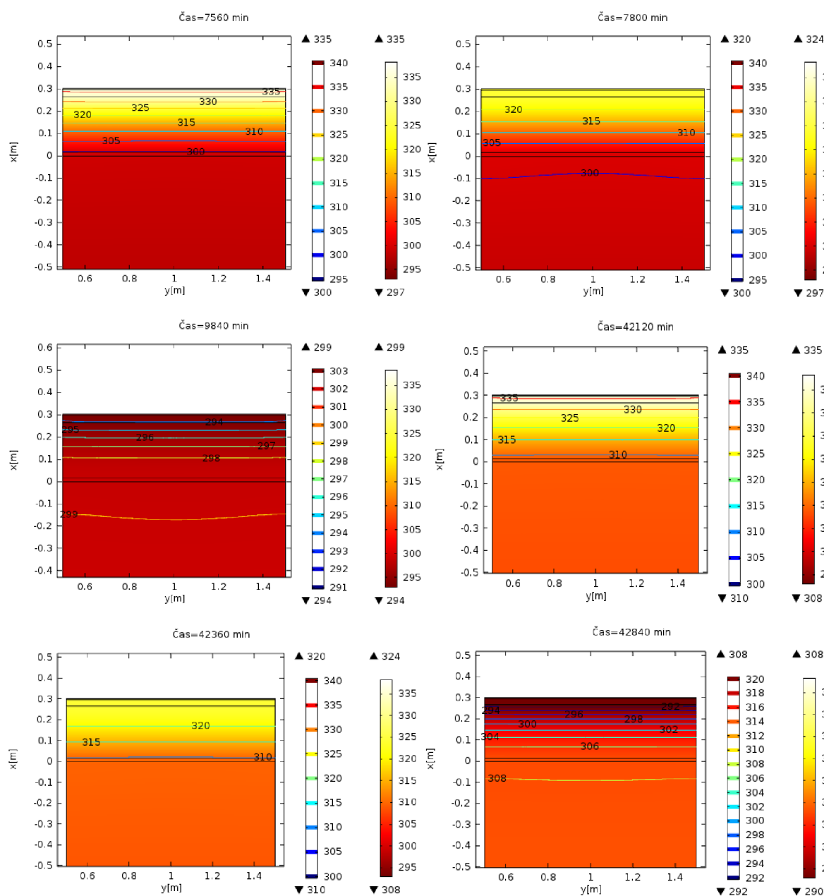
Obr. 26 Teplotní profil střešního pláště a části přilehlého interiéru v časech od počátku simulace 0h, 1h, 3h, 6h, 10h, 18h, 30h, 34h, 126h, 130h 164h (cca 1 týden), 702h (29 dní a 6h), 706h (29 dní a 10h) a 714h (29dní a 18h), stupnice jsou uvedeny v Kelvinech
