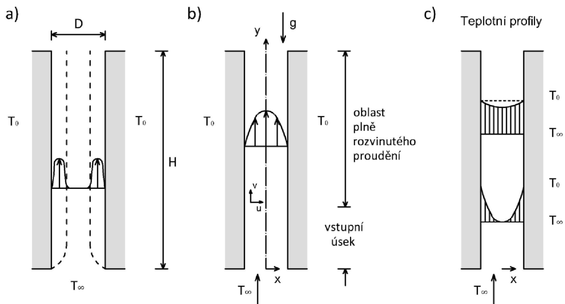
Obr. 11 Větraná vzduchová vrstva mezi dvěma vyhříványými konstrukcemi: a) vzdálenost konstrukcí D > 2 \delta_T ; b) vzdálenost konstrukcí D \leq 2 \delta_T ; c) teplotní profil v dutině [44]
