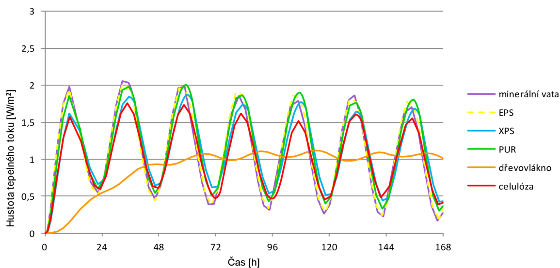
Obr. 30 Vliv materiálu tepelné izolace: Tepelné toky na lici stropního podhledu v periodě 7 dní
