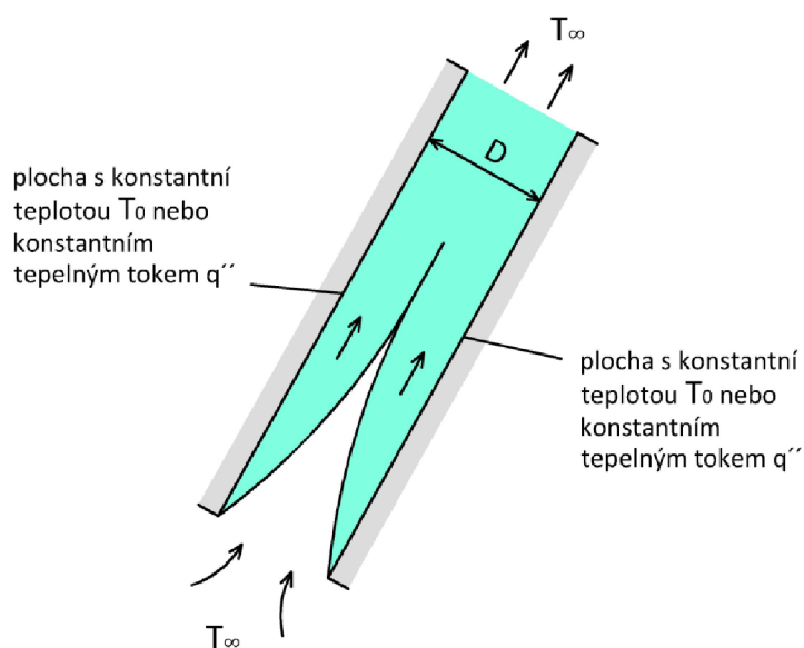
Obr. 12 Vývin mezních vrstev ve větrané dutině [39]
