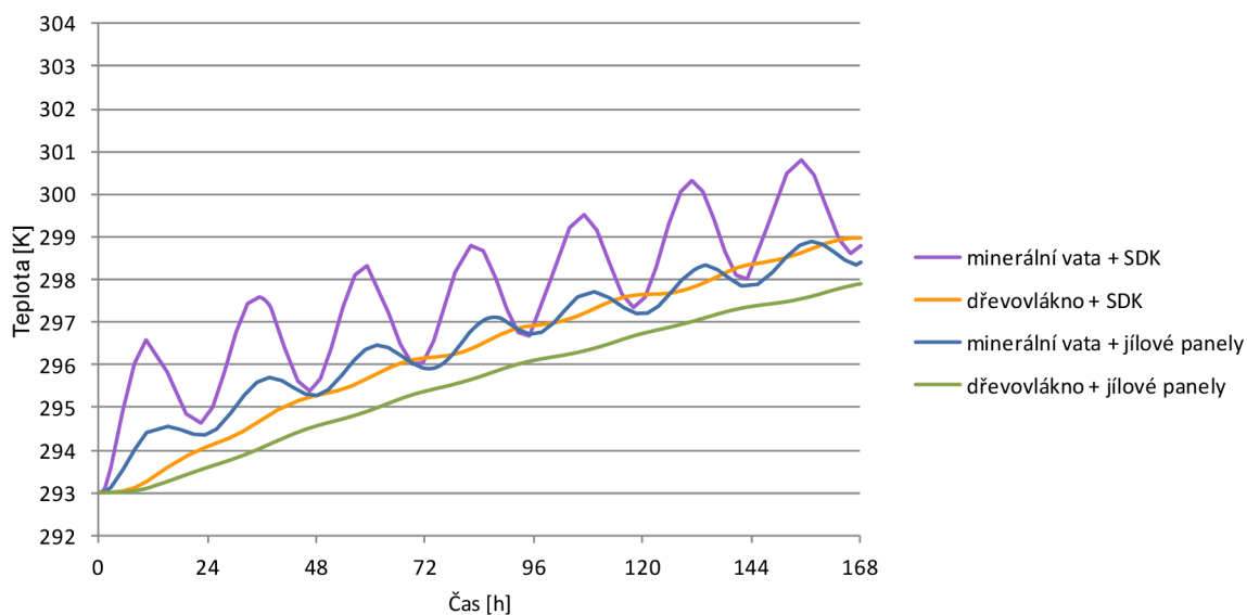
Obr. 33 Vliv kombinace materiálů tepelné izolace a podhledu: Teploty na lici stropního podhledu v periodě 7 dní
