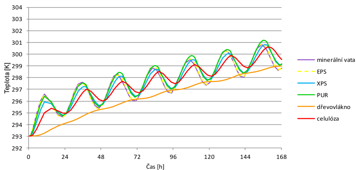
Obr. 29 Vliv materiálu tepelné izolace: Teploty na lici stropního podhledu v periodě 7 dní
