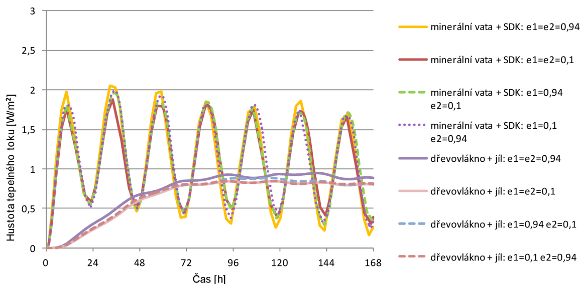
Obr. 36 Vliv reflexních povrchů: Tepelné toky na lici stropního podhledu v periodě 7 dní
