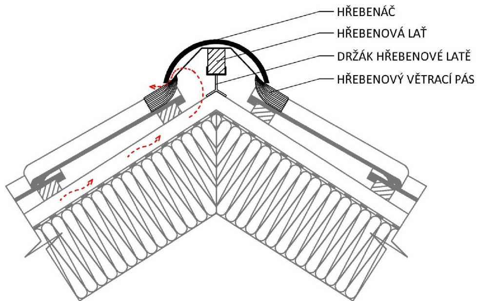
Obr. 88 Současné řešení detailu střešního hřebene
