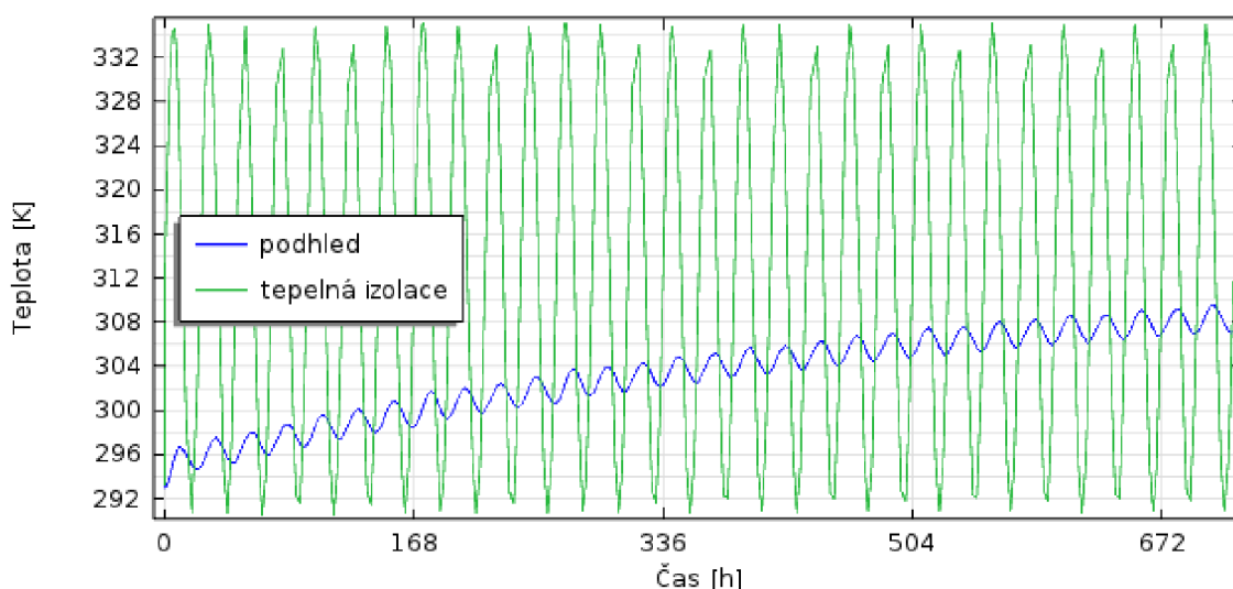
Obr. 28 Průběh povrchových teplot ve střešním plášti pasivní budovy, materiálové řešení s minerální vatou a sádkartonem v měsíčním horizontu
