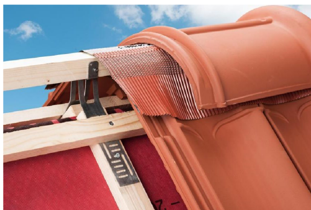
Obr. 84 Hřebenový větrací pás celohliníkový s perforací [70]
