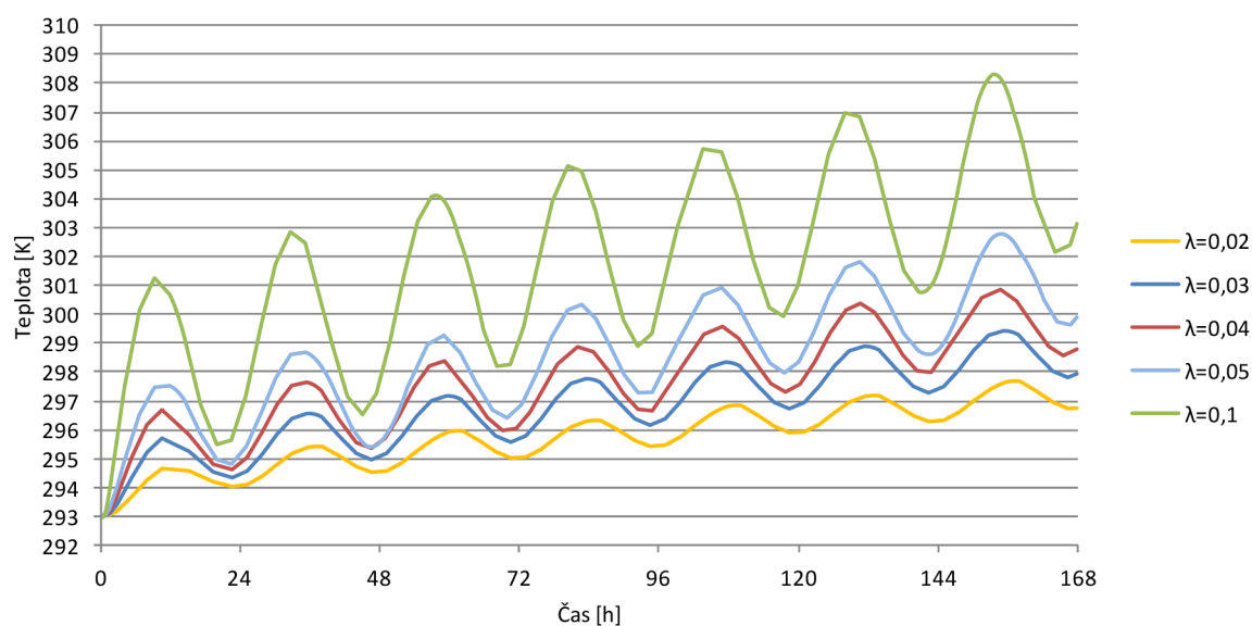
Obr. 51 Vliv součinitele tepelné vodivosti na teplotu líce stropního podhledu – teploty
