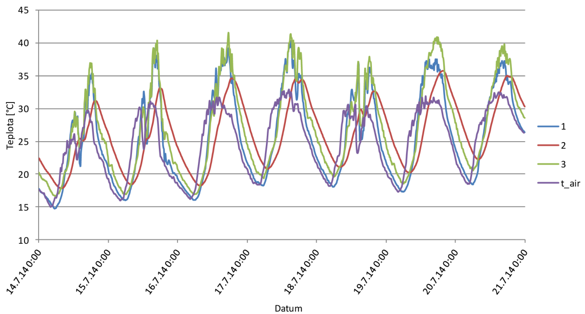
Obr. 44 Rozložení teplot v modelu střešního pláště – pole D (lisovaná sláma + reflexní fólie)
