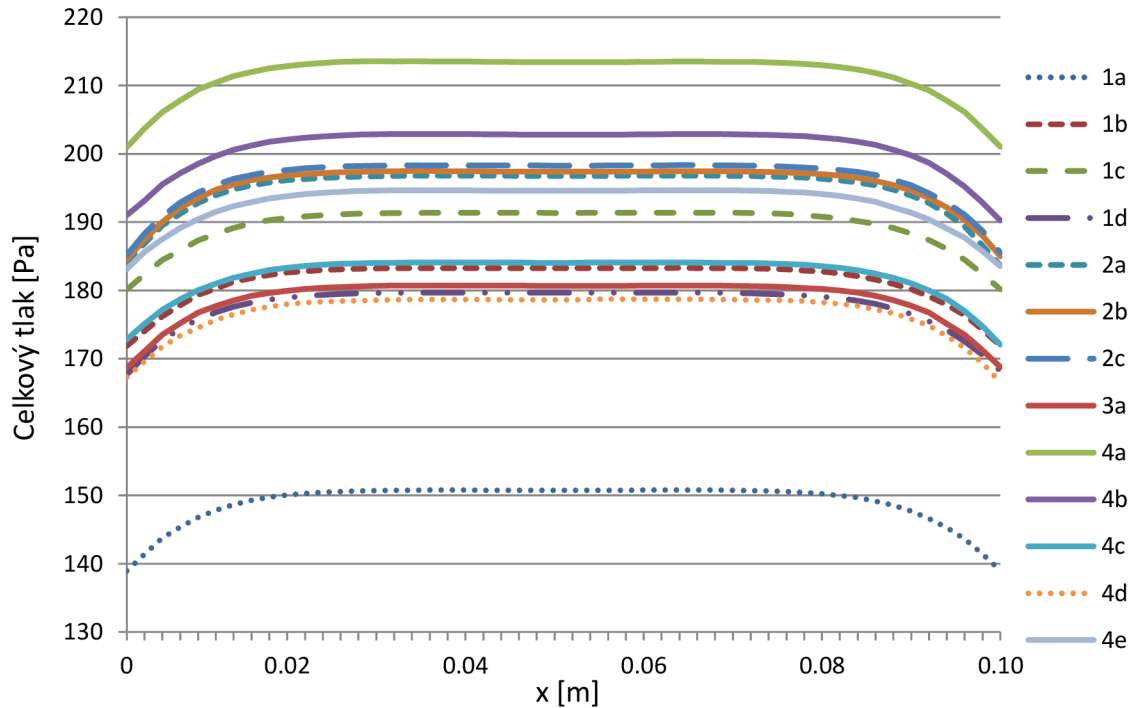
Obr. 69 Celkový tlak 20 mm před mřížkami [73]
