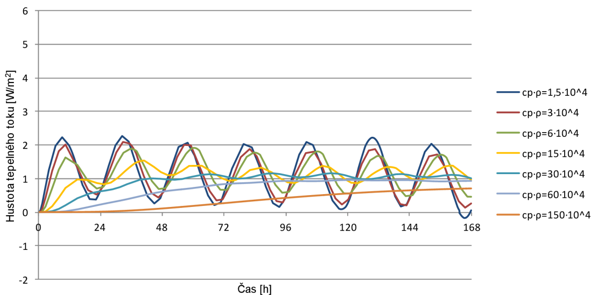
Obr. 54 Vliv objemové tepelné kapacity na teplotu líce stropního pohledu – tepelné toky
