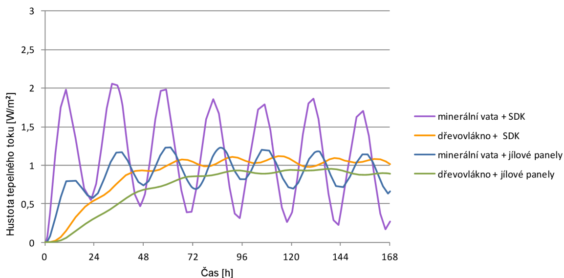
Obr. 34 Vliv kombinace materiálů tepelné izolace a podhledu: Tepelné toky na lici stropního podhledu v periodě 7 dní
