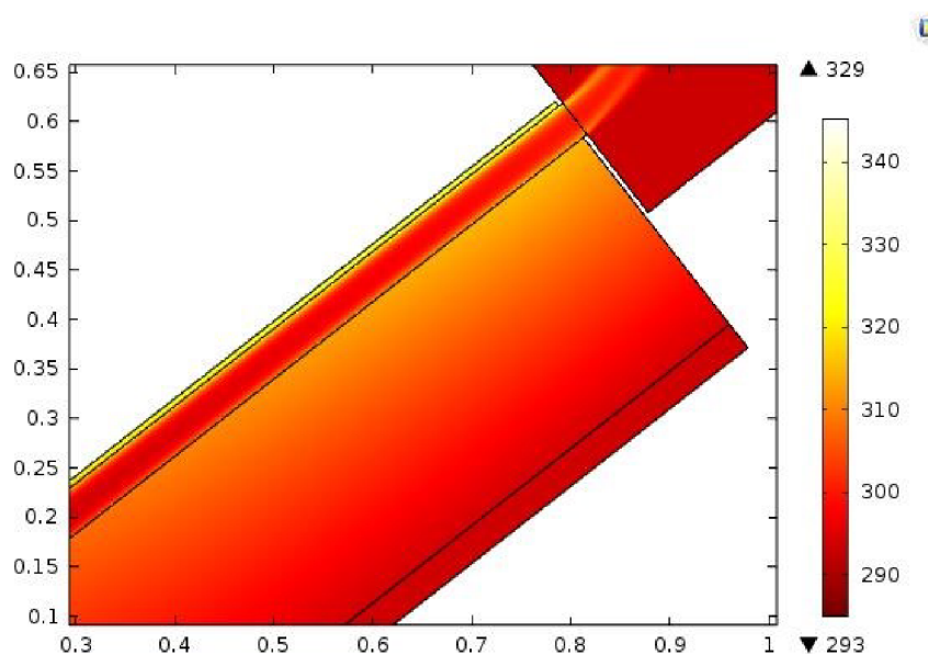
Obr. 58 Rozložení teplot ve střešním plášti – vysoká emisivita povrchů ve větrané dutině \epsilon_1 = \epsilon_2 = 0,94
