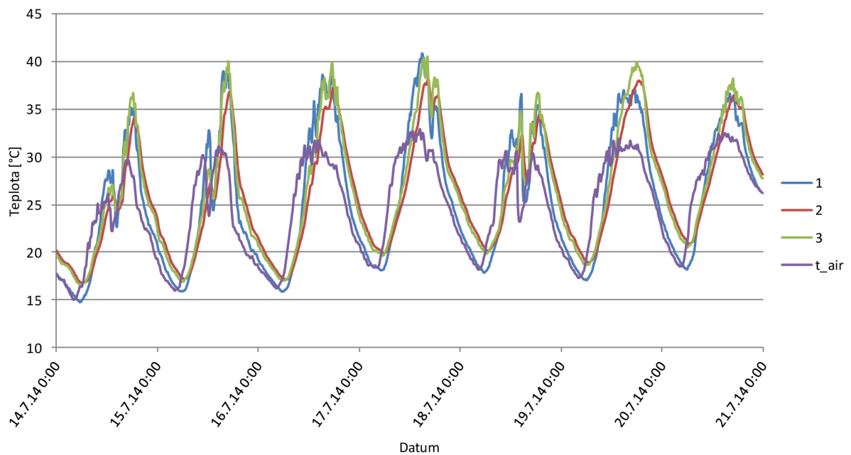
Obr. 42 Rozložení teplot v modelu střešního pláště – pole B (SDK + reflexní fólie)
