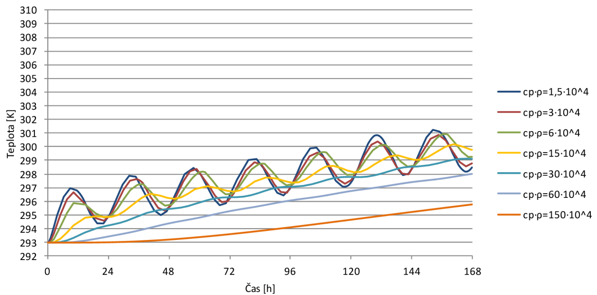
Obr. 53 Vliv objemové tepelné kapacity na teplotu líce stropního pohledu – teploty
