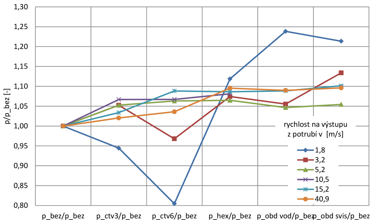
Obr. 72 Poměr tlaku v potrubí pro mřížky vztažený k tlaku v potrubí bez mřížky
