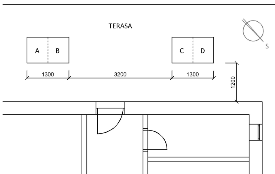
Obr. 23 Schéma terasy s umístěním modelů
