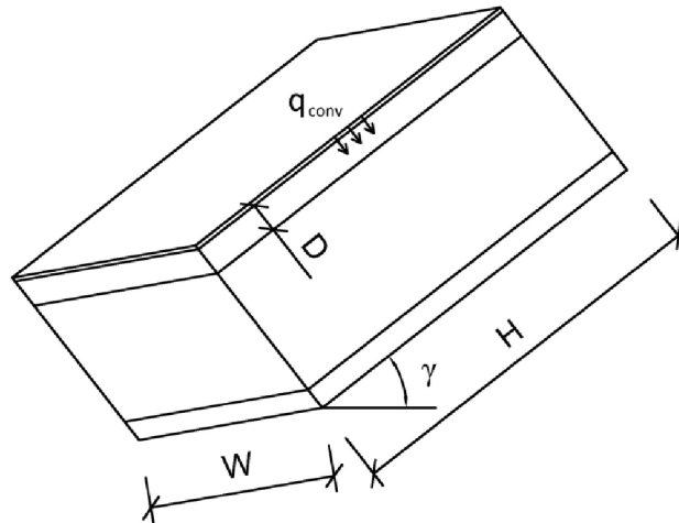
Obr. 8 Schéma větraného střešního pláště
