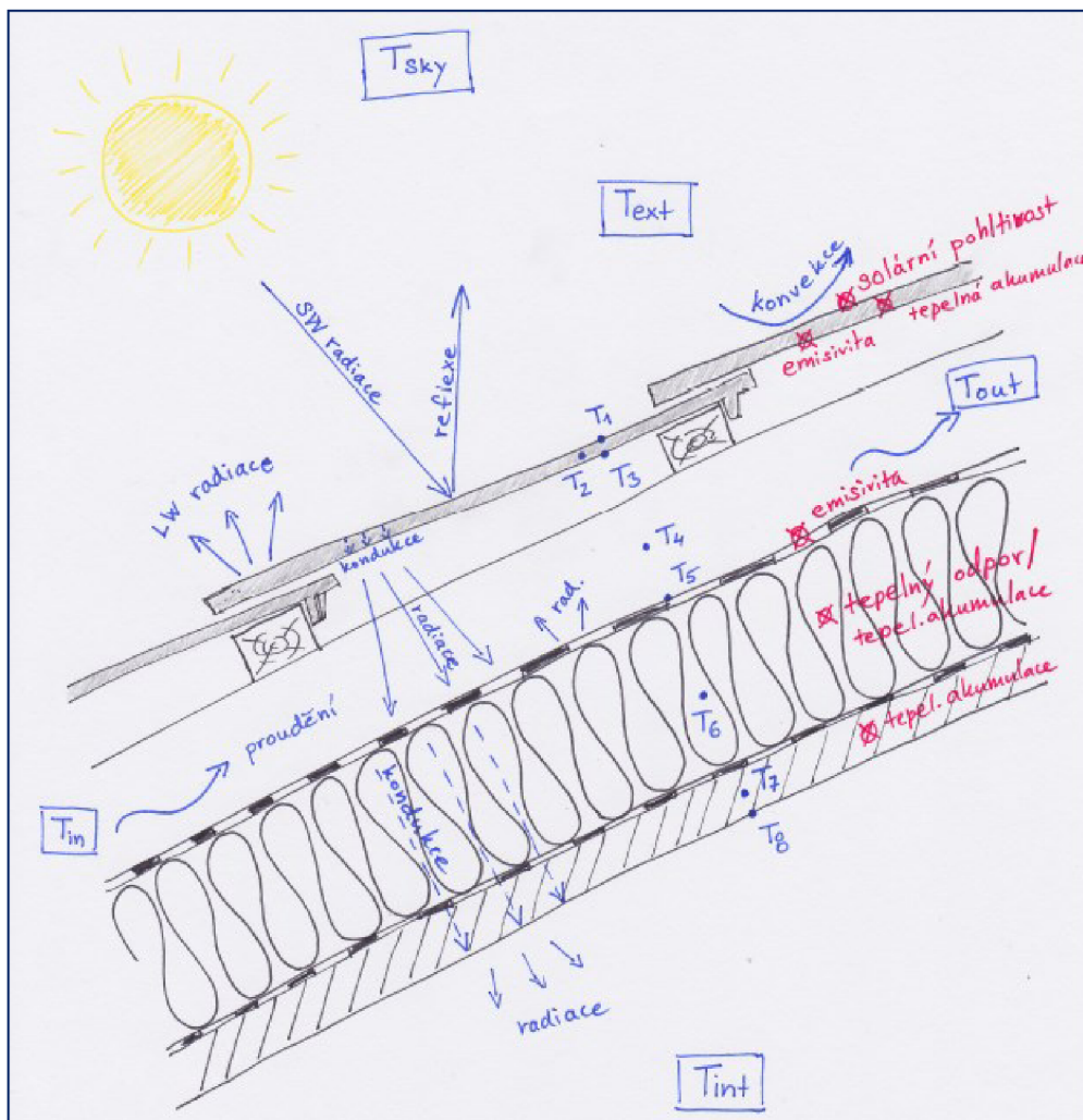
Obr. 14 Distribuce tepla ve střešním plášti
