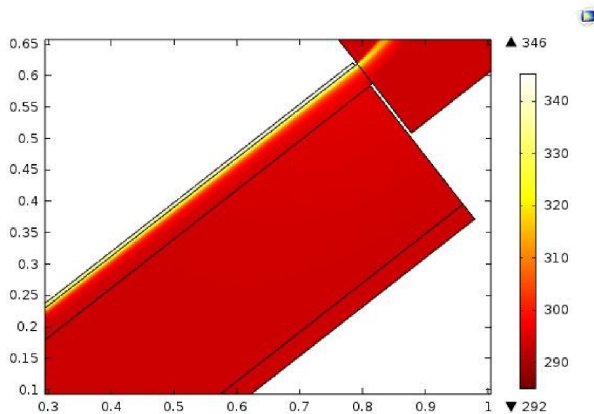
Obr. 57 Rozložení teplot ve střešním plášti – nízká emisivita povrchů ve větrané dutině (bez vlivu radiační složky)[72]
