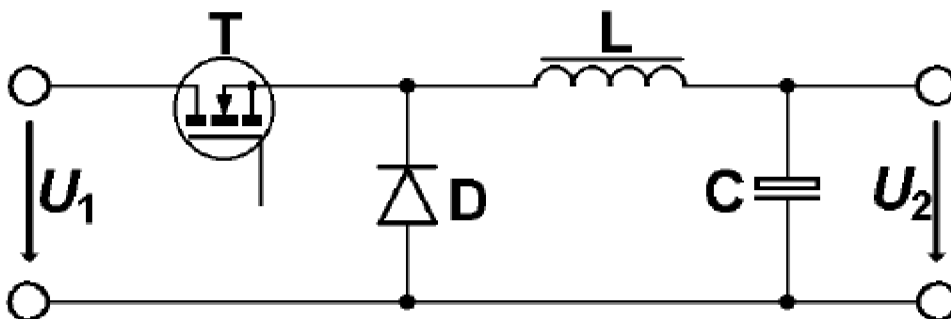
Obr. 2 Znižujúci menič [5]
