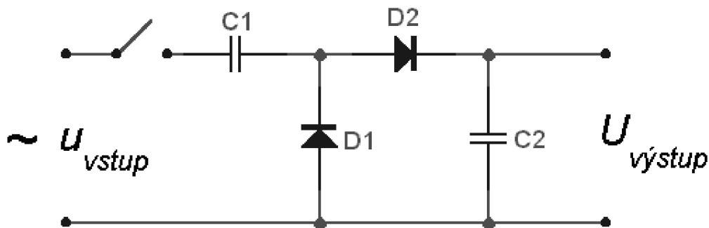
Obr. 5 Zdvojovač napätia [5]
