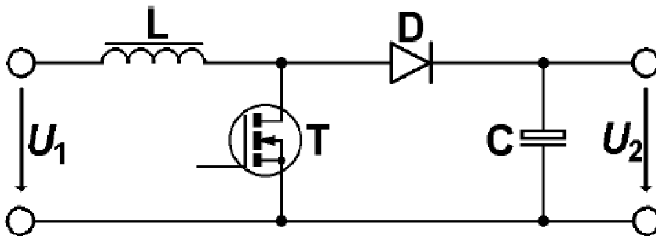
Obr. 3 Zvyšujúci menič [5]
