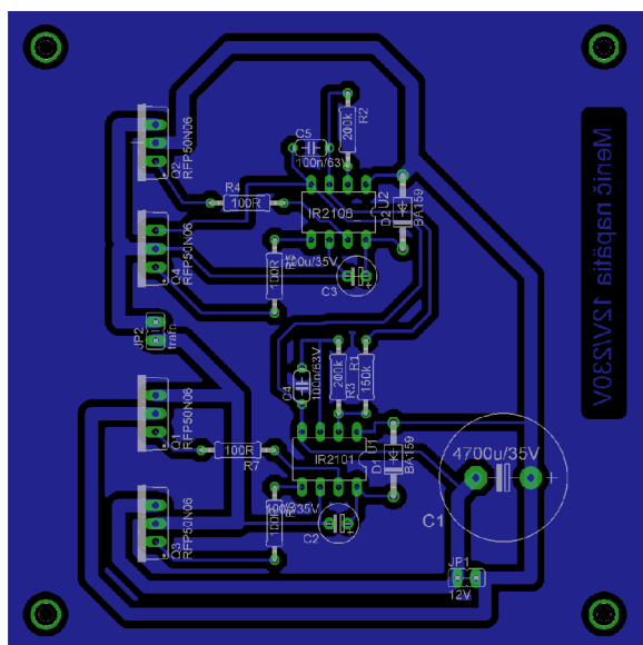
Obr. 16 Osadzovací výkres
