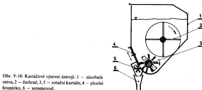
Obrázek 1.2 Kartáčkové secí ústrojí (Neubauer et al., 1989)
