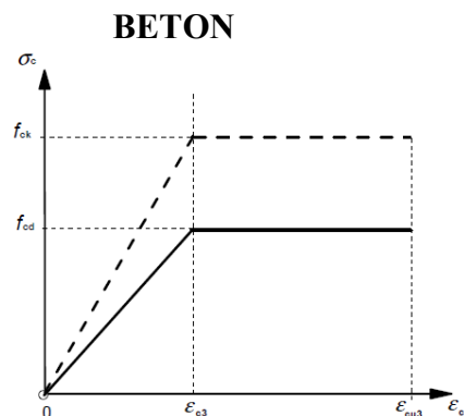
Obrázek 3.4 – Bilineární pracovní diagram
