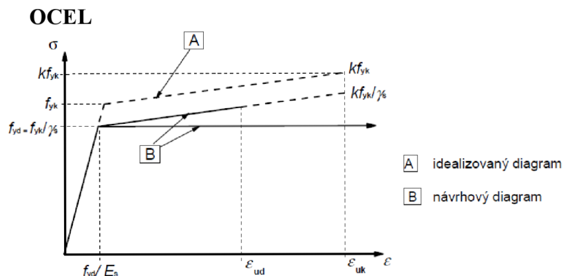
Obrázek 3.8 – Schéma pracovních diagramů betonářské oceli (pro tah i tlak)
