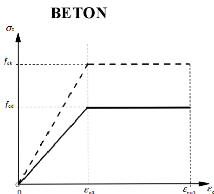
Obrázek 3.4 – Bilineární pracovní diagram
