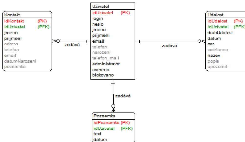
Obrázek 2.2 – ER diagram
