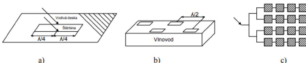
Obrázek 5 a) Štěrbínová anténa b) Soustava štěrbin ve vlnovodu c) Mikropásková
