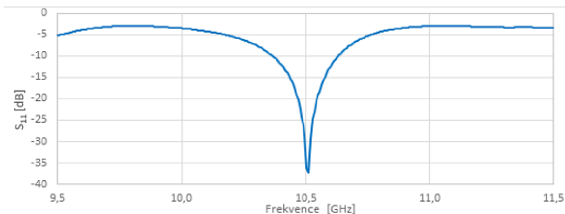
Obrázek 19 Činitel odrazu SIW štěrbinové antény
