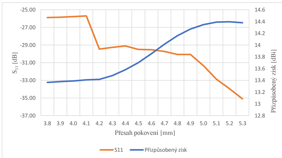
Obrázek 41 Vliv přesahu pokovení na zisk a činitel odrazu
