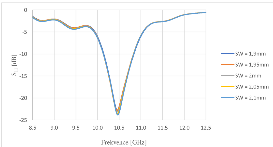
Obrázek 12 Simulace změny šířky štěrbiny vlnovodné štěrbinové antény
