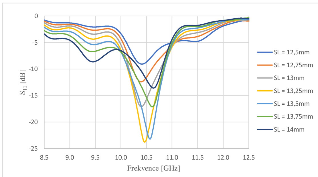
Obrázek 11 Simulace změny délky štěrbiny vlnovodné štěrbinové antény
