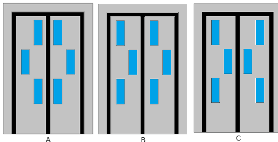
Obrázek 25 Varianty vyzařovací části antény
