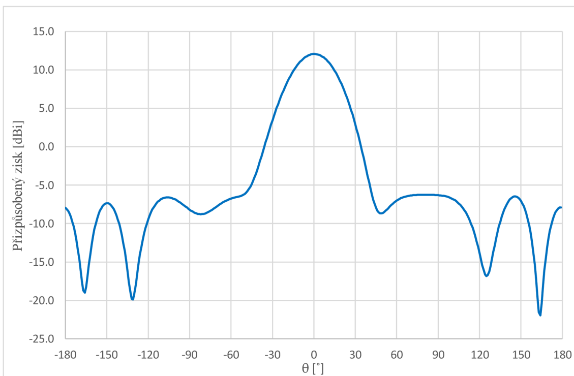
Obrázek 48 Směrová charakteristika 3x2 anténní řady s mikropáskovým přechodem v rovině E
