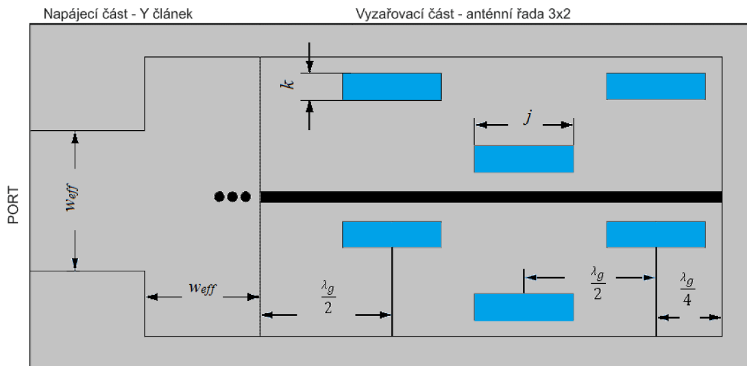
Obrázek 26 Anténní řada 3x2 s pevnými stěnami
