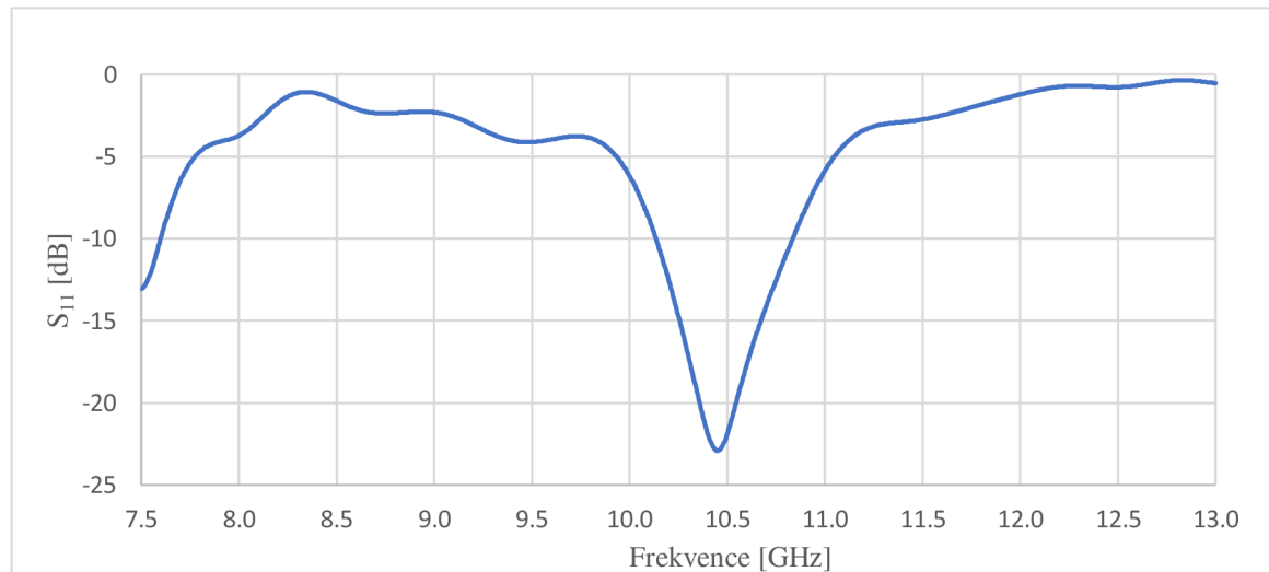
Obrázek 10 Činitel odrazu vlnovodné štěrbinové antény
