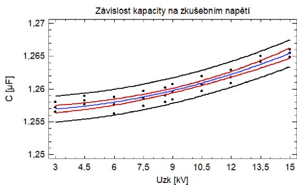
Graf 31A – Závislost kapacity na zkušební napětí, měřeno v roce 2019
