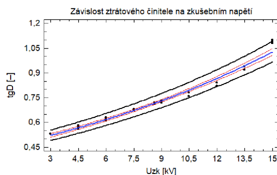
Graf 4A – Závislost ztrátového činitele na zkušební napětí, měřeno v roce 2006
