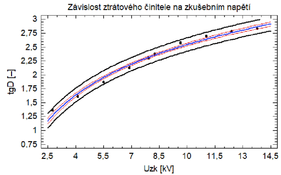
Graf 22D – Závislost ztrátového činitele na zkušebním napětí, měřeno v roce 2015
