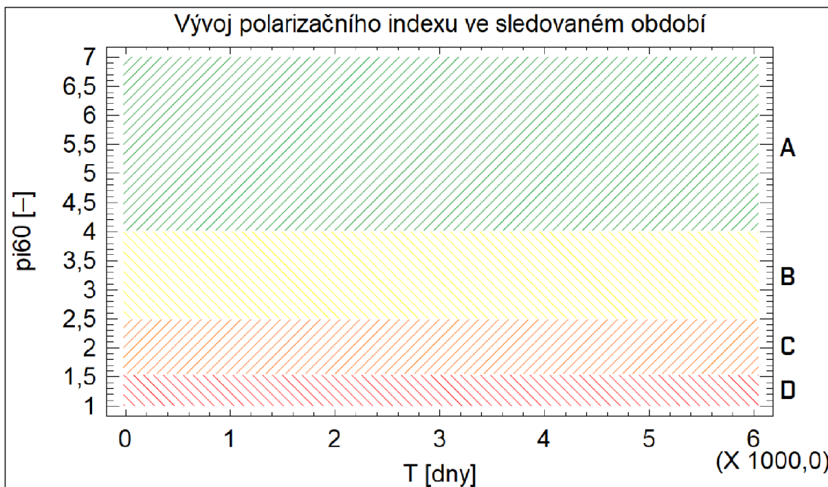
Obr. č. 4: Zobrazení polí škál A – D pro hodnocení \pi_{i60}
