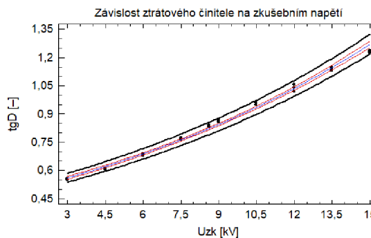
Graf 32B – Závislost ztrátového činitele na zkušební napětí, měřeno v roce 2018
