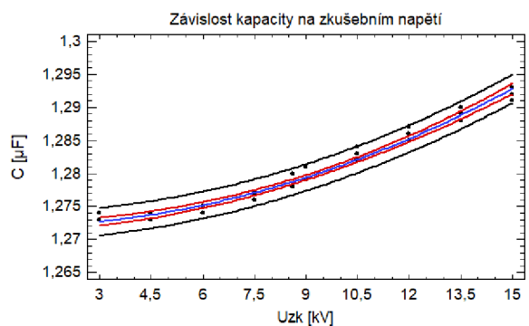
Graf 7A – Závislost kapacity na zkušební napětí, měřeno v roce 2008
