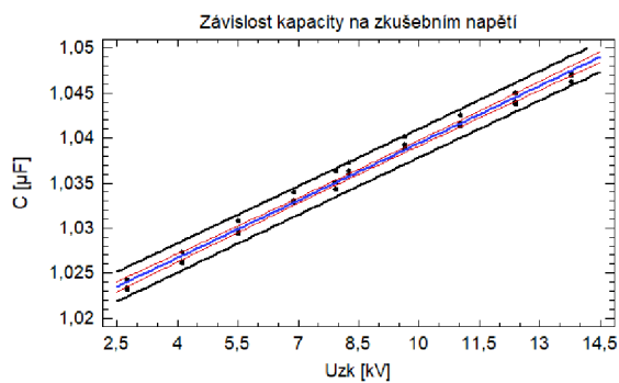
Graf 7C – Závislost kapacity na zkušebním napětí, měřeno v roce 2010 poprvé
