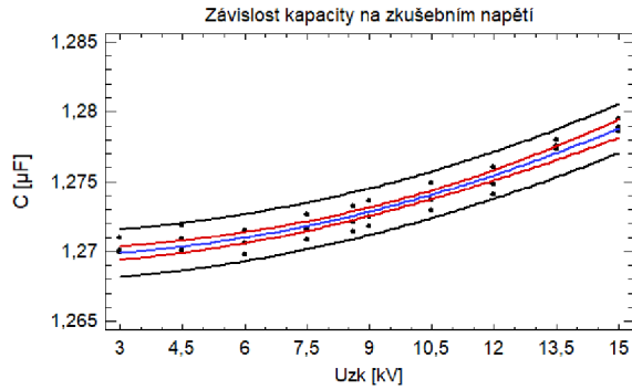
Graf 25A – Závislost kapacity na zkušební napětí, měřeno v roce 2016
