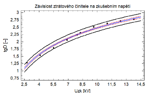
Graf 24D – Závislost ztrátového činitele na zkušebním napětí, měřeno v roce 2016
