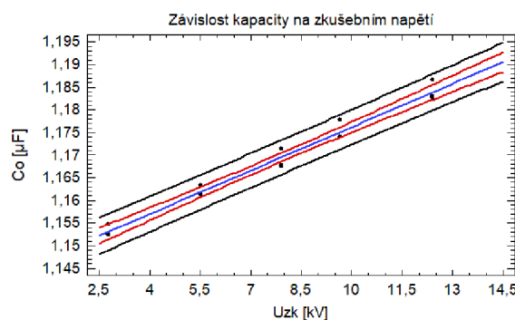
b) Regresní křivka s optimalizovaným počtem měření (polovičním)
