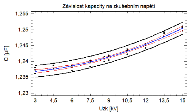
Graf 37B – Závislost kapacity na zkušební napětí, měřeno v roce 2021
