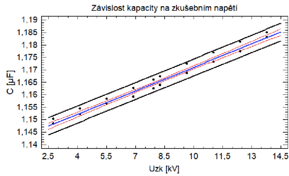
Graf 21D – Závislost kapacity na zkušebním napětí, měřeno v roce 2015
