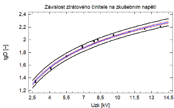
Graf 8C – Závislost ztrátového činitele na zkušebním napětí, měřeno v roce 2010 poprvé
