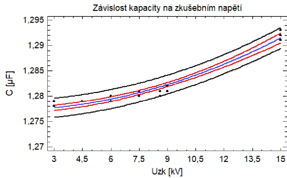
Graf 9A – Závislost kapacity na zkušební napětí, měřeno v roce 2009
