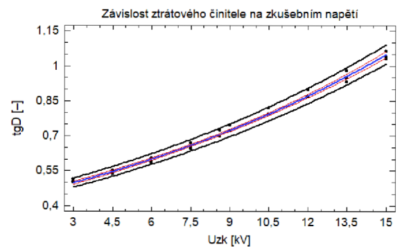
Graf 36A – Závislost ztrátového činitele na zkušební napětí, měřeno v roce 2021
