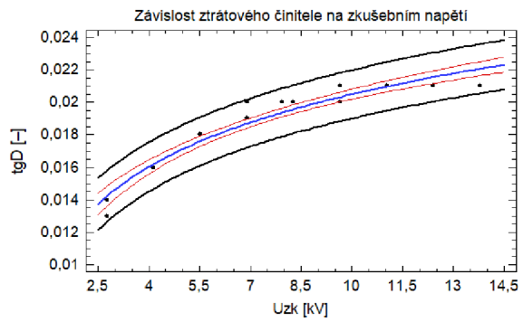
Graf 6C – Závislost ztrátového činitele na zkušebním napětí, měřeno v roce 2009
