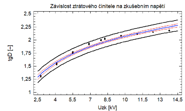
Graf 20C – Závislost ztrátového činitele na zkušebním napětí, měřeno v roce 2015
