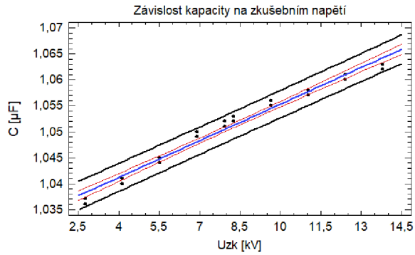
Graf 5C – Závislost kapacity na zkušebním napětí, měřeno v roce 2009
