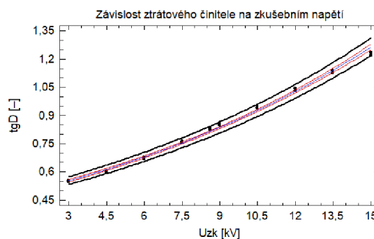
Graf 30B – Závislost ztrátového činitele na zkušební napětí, měřeno v roce 2017
