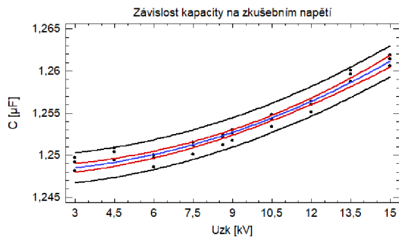
Graf 29B – Závislost kapacity na zkušební napětí, měřeno v roce 2017
