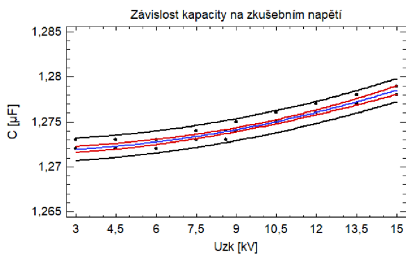
Graf 5A – Závislost kapacity na zkušební napětí, měřeno v roce 2007
