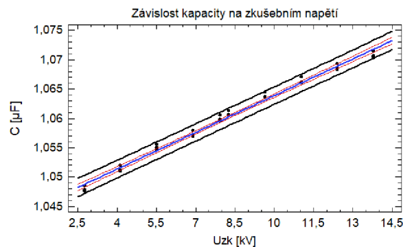
Graf 19C – Závislost kapacity na zkušebním napětí, měřeno v roce 2015
