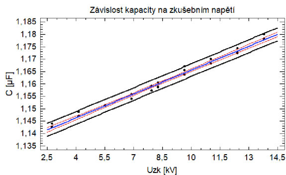
Graf 23D – Závislost kapacity na zkušebním napětí, měřeno v roce 2016
