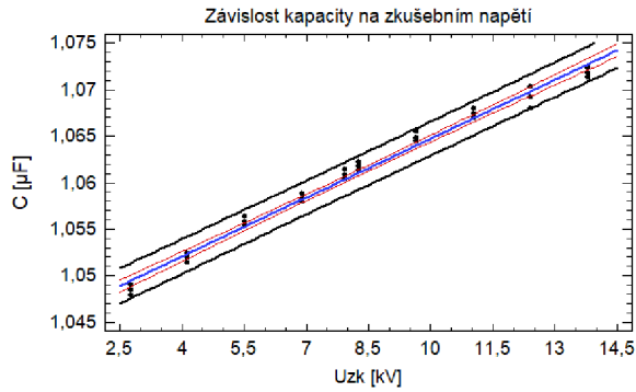
Graf 17C – Závislost kapacity na zkušebním napětí, měřeno v roce 2014
