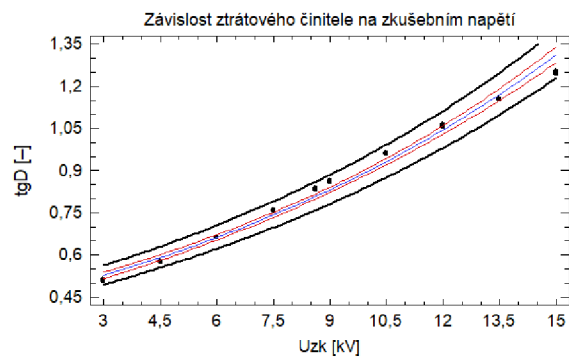
Graf 38B – Závislost ztrátového činitele na zkušební napětí, měřeno v roce 2021
