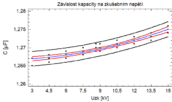
Graf 13B – Závislost kapacity na zkušební napětí, měřeno v roce 2009
