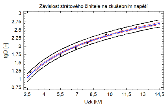
Graf 2D – Závislost ztrátového činitele na zkušebním napětí, měřeno v roce 2005
