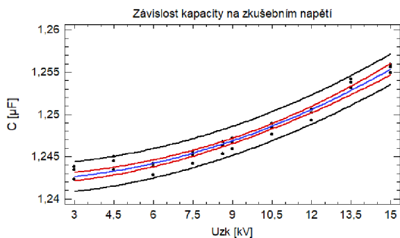
Graf 31B – Závislost kapacity na zkušební napětí, měřeno v roce 2018
