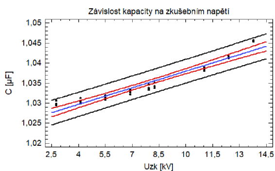
Graf 3C – Závislost kapacity na zkušební napětí, měřeno v roce 2008
