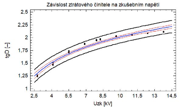
Graf 18C – Závislost ztrátového činitele na zkušebním napětí, měřeno v roce 2014
