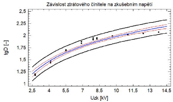
Graf 30C – Závislost ztrátového činitele na zkušební napětí, měřeno v roce 2020
