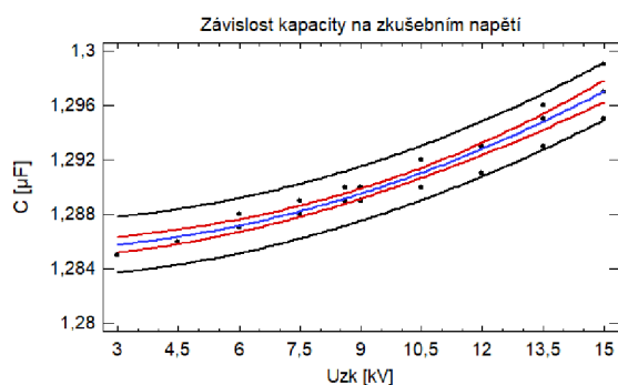
Graf 3A – Závislost kapacity na zkušební napětí, měřeno v roce 2006
