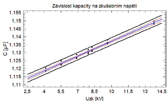
Graf 1D – Závislost kapacity na zkušebním napětí, měřeno v roce 2005
