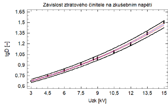
Graf 14B – Závislost ztrátového činitele na zkušební napětí, měřeno v roce 2009
