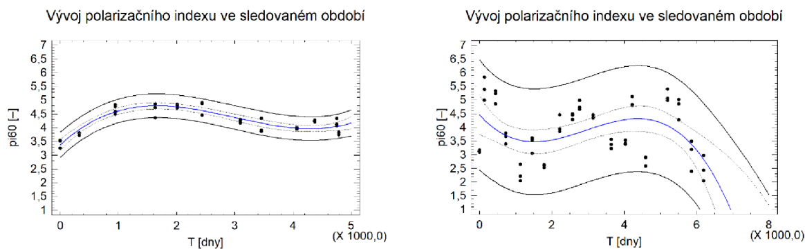
b) Regresní křivka polarizačního indexu generátoru G4
