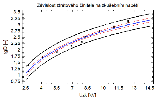
Graf 4D – Závislost ztrátového činitele na zkušebním napětí, měřeno v roce 2006
