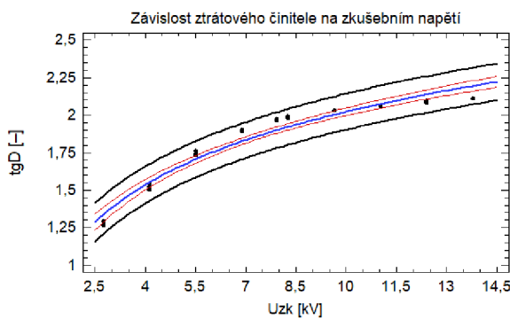
Graf 16C – Závislost ztrátového činitele na zkušební napětí, měřeno v roce 2013
