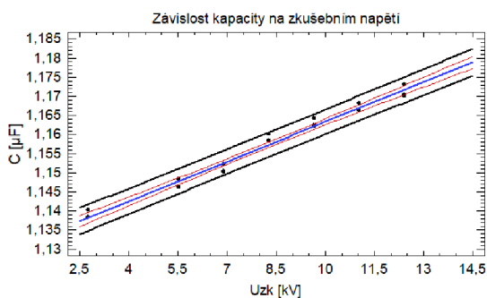
Graf 3D – Závislost kapacity na zkušebním napětí, měřeno v roce 2006
