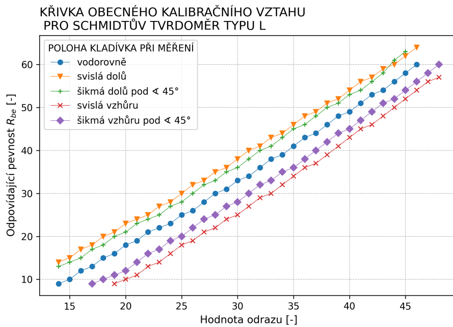
Obr. 1.5: Křivky pro Schmidtvův tvrdoměr typu L sestavené podle normou uvedené tabulky [2]
