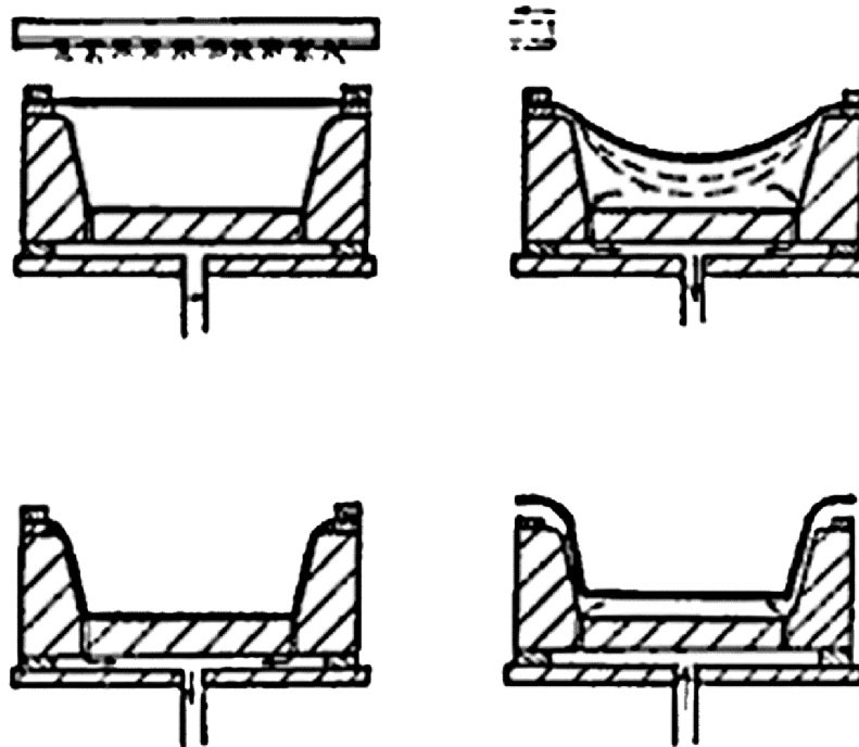
Obrázek 3.8: Schéma pozitivního, negativního a kombinovaného tvarování (techportal.cz, 2022)
