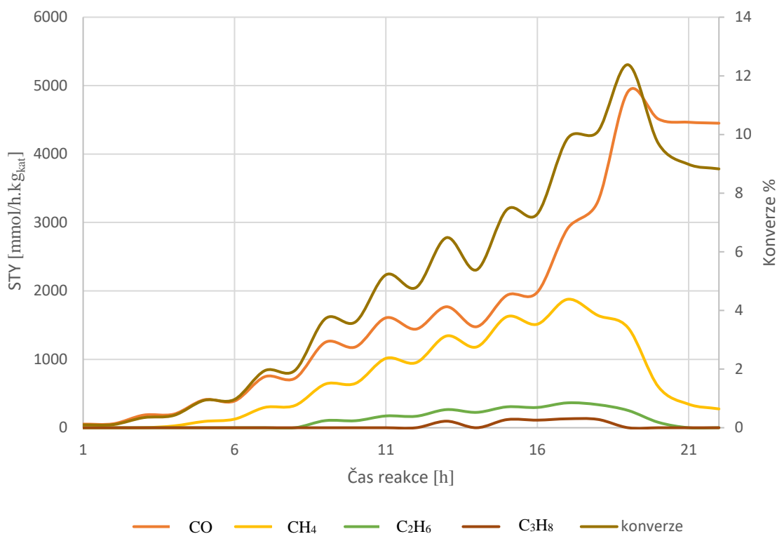
Obř. 19: Grafická závislost množství produktů (STY) a konverze na čase reakce pro kompozit Ag@TiO 2 s 10% obsahem mědi
