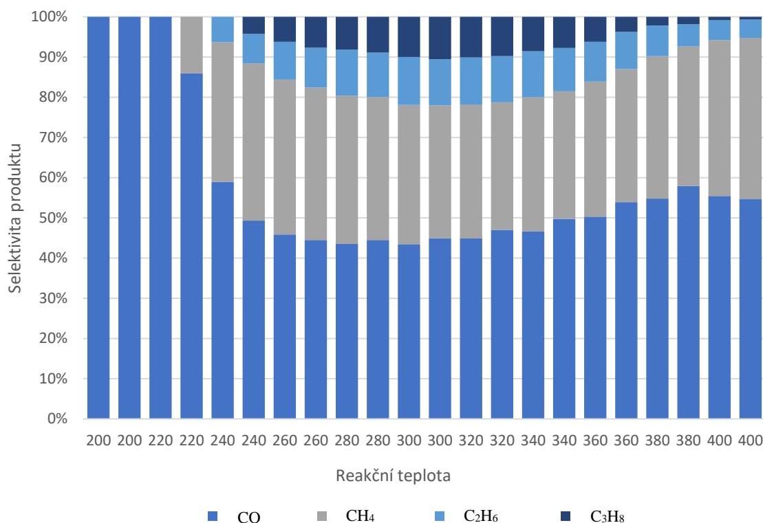
Obr. 17: Závislost reakční teploty na selektivě produktu pro oxid uhelnatý, methan, ethan a propan pro kompozit Cu@Fe 2 O 3 s 10% obsahem Cu
