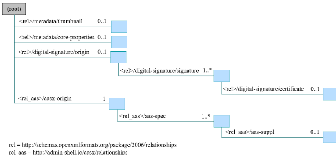
Obr. 1.7: Diagramová ukázka typů vztahů v souboru AASX [10]
