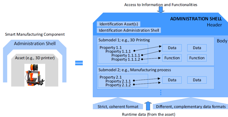
Obr. 1.1: Struktura AAS [7]
