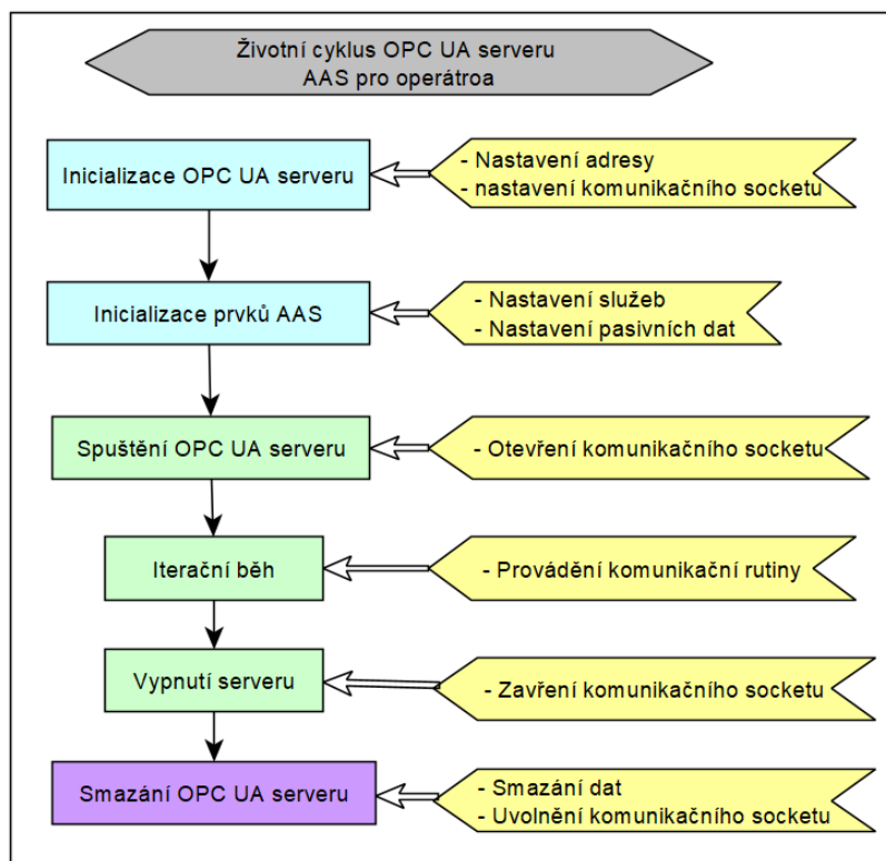
Obr. 2.15: Digram životního cyklu OPC UA v AAS pro operátora
