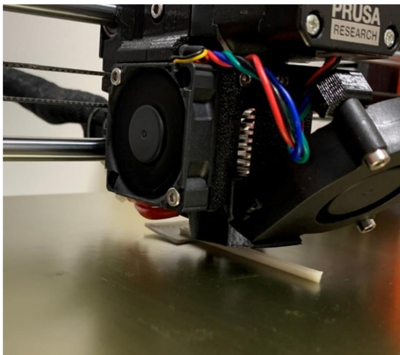
Obrázek 12 Warping testovacího tělesa vzorku G_80/20-23
