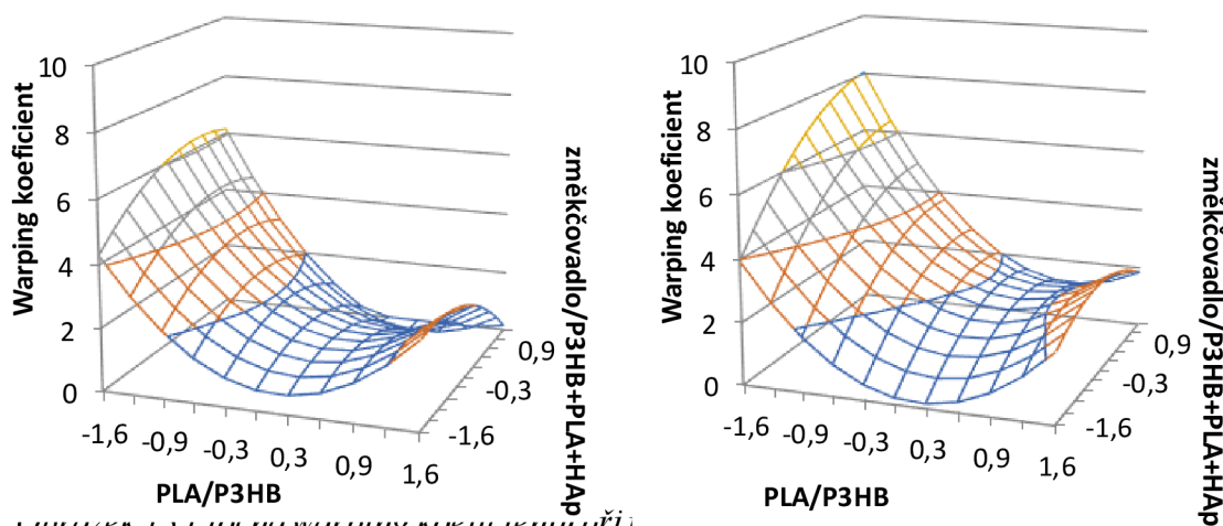
Obrázek 13 Dvě plochy warping koeficientu při nejnižším a nejvyšším testovaném množství HAp (vpravo)
