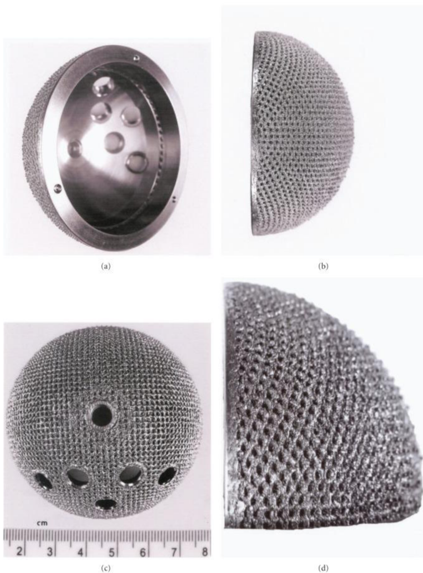
Obrázek 3 Titanový implantát pro náhradu kyčelního kloubu (10)
