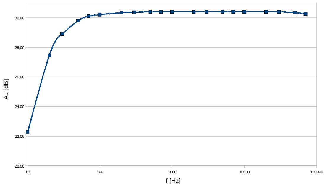
Obr. 12 Modulová frekvenční charakteristika výkonového zesilovače pro kanál 1
