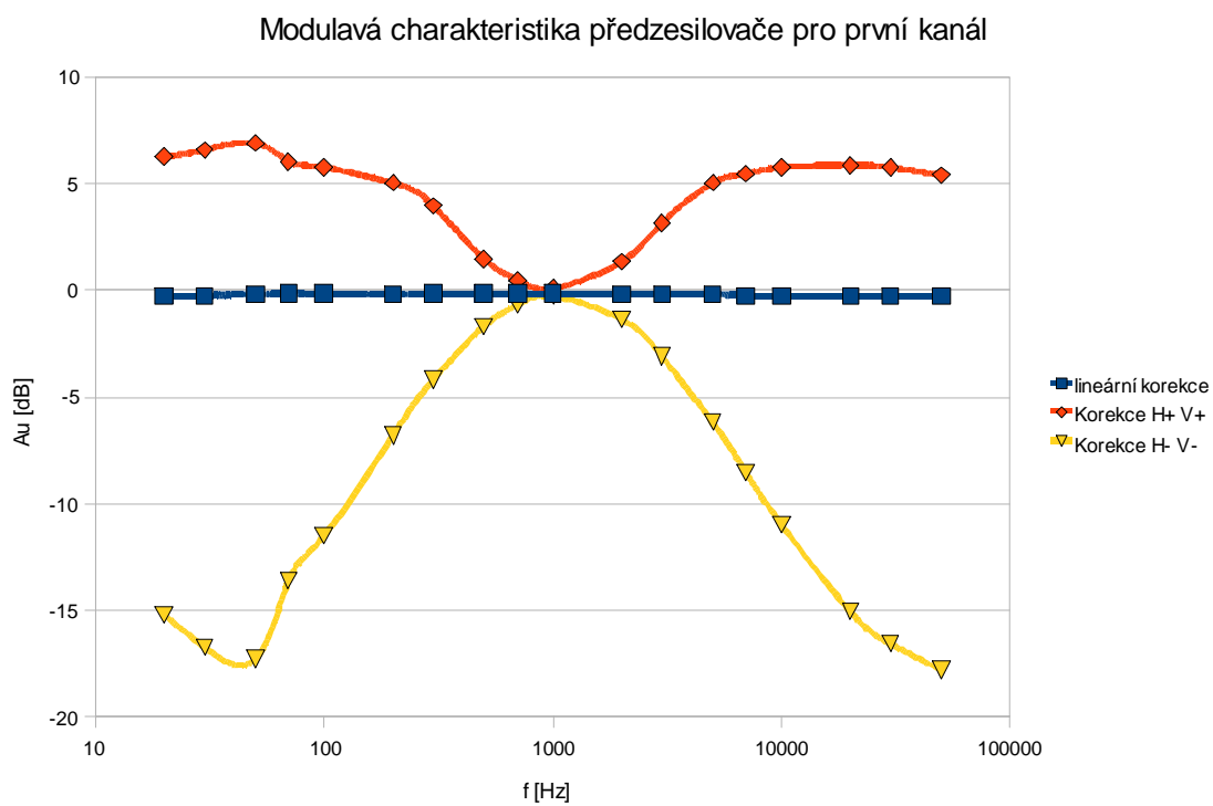
Obr. 10 Modulová kmitočtová charakteristika předzesilovače pro kanál 1
