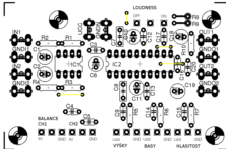
Obrázek VII Osazovací plán korekčního předzesilovače
