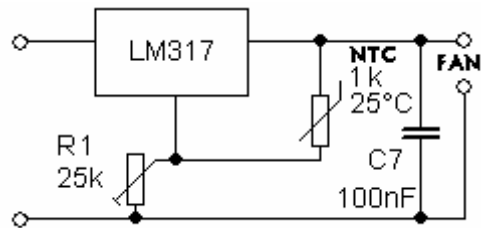
Obr. 9 Regulace otáček ventilátoru
