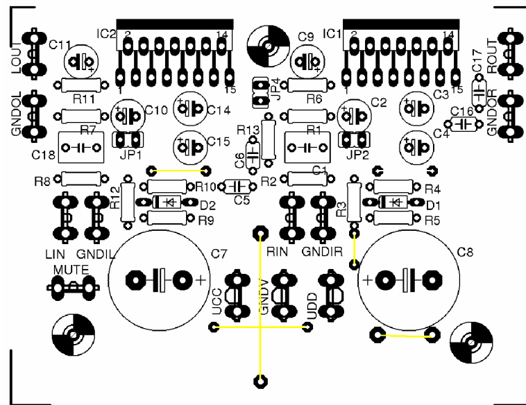
Obrázek VIII Osazovací plán výkonového zesilovače pro dva kanály
