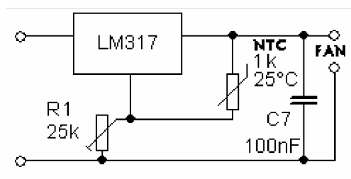
Obr. 9 Regulace otáček ventilátoru
