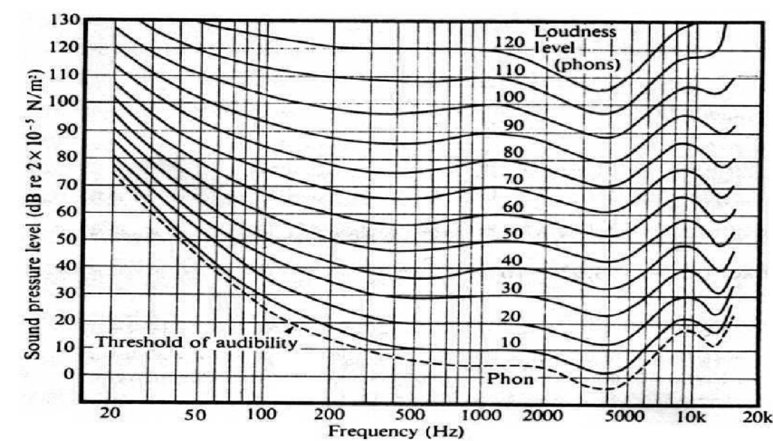
Obr. 2 Fletcher-Munsonovy křivky (převzato z [1])
