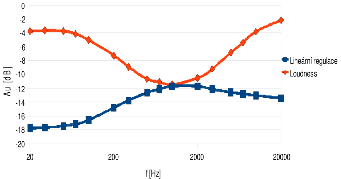
Obr. 11 Frekvenční závislost regulace hlasitosti korekčního předzesilovače pro kanál 1
