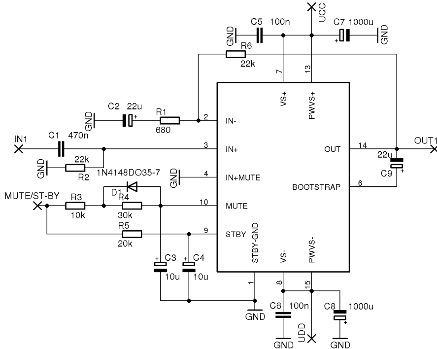
Obr. 6 Schéma zapojení jednoho kanálu výkonového zesilovače (převzato z [5] )
