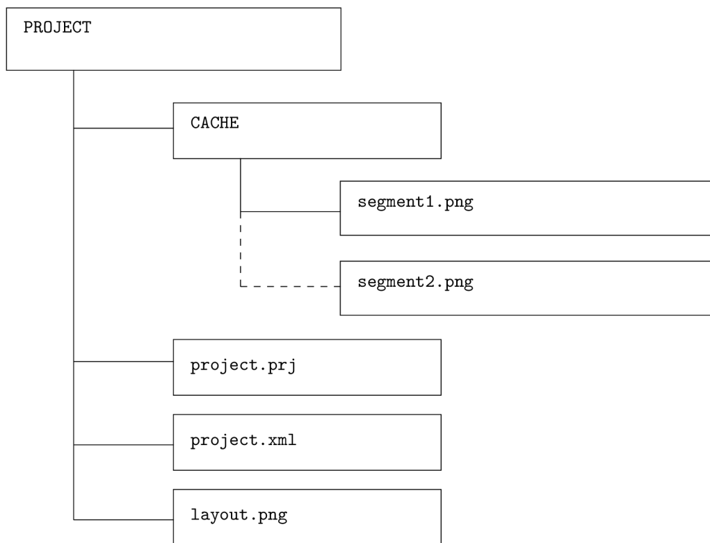
Obrázek 3.20: Hierarchie projektu
