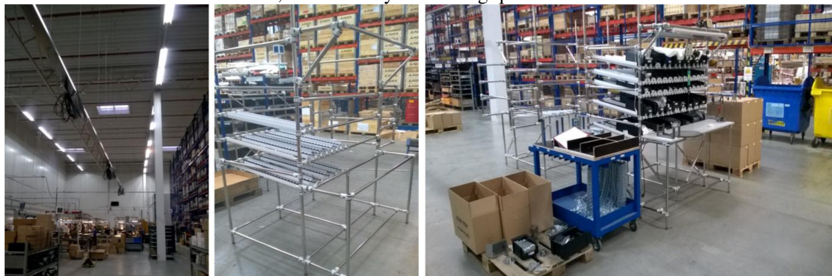
Obrázek 14 Nová elektroinstalace, modulární systém Trilogiq
