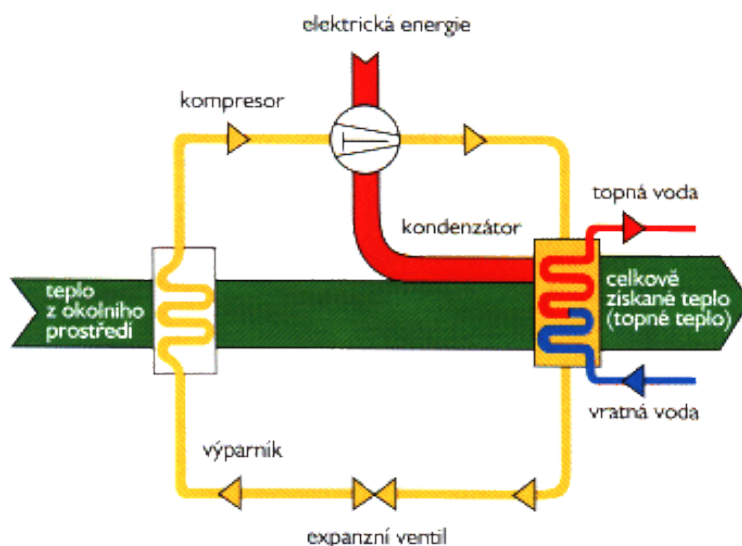
Obr. 6 Tepelné čerpadlo [4]
