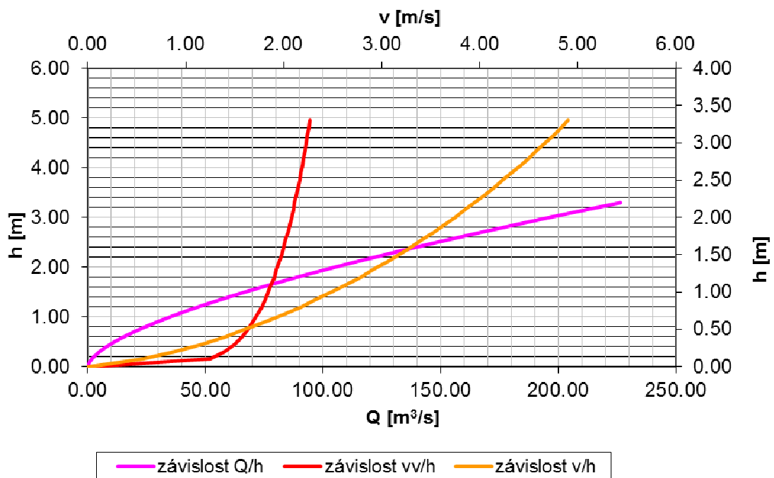
Obr.22 Graf závislosti výšky na rychlosti a průtoku pro profil 1 a efektivní zrna 30mm
