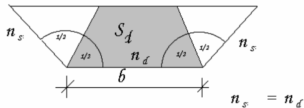
Obr.18 Schéma koryta v přímé
