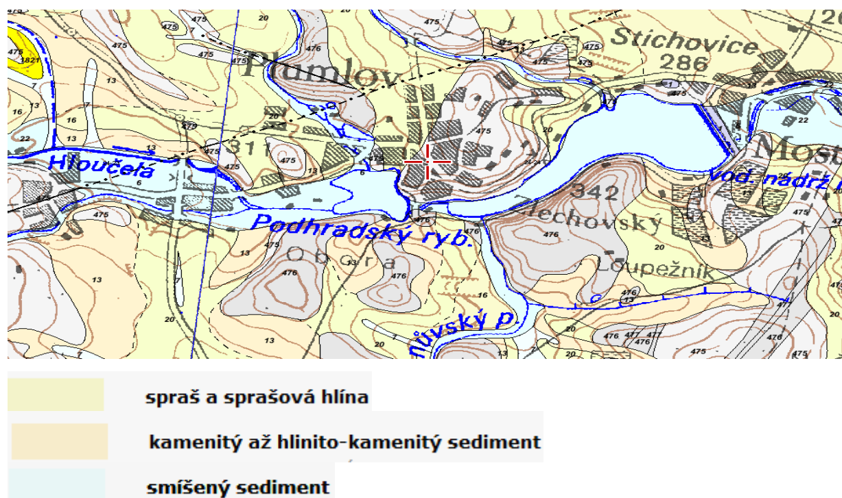
Obr.3 Geologická situace
