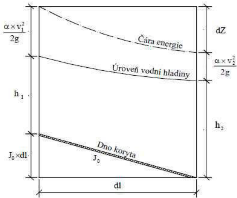
Obr.20 Schématické znázornění úseku pro odvození Bernoulliovi rovnice
