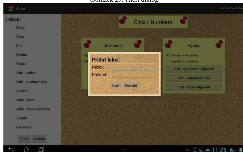
Obrázek 30: Vlastní dialog
