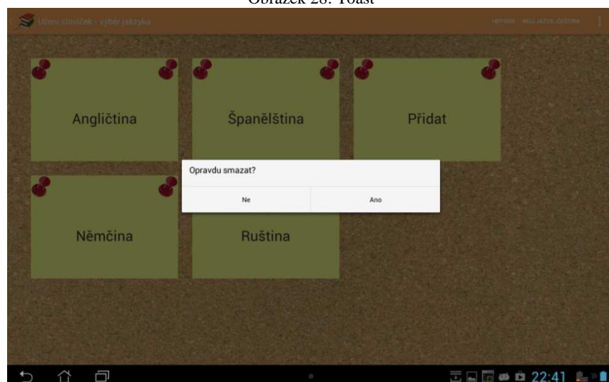
Obrázek 29: Alert dialog
