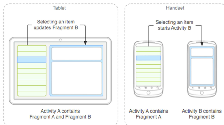
Obrázek 3: Logika fragmentu
