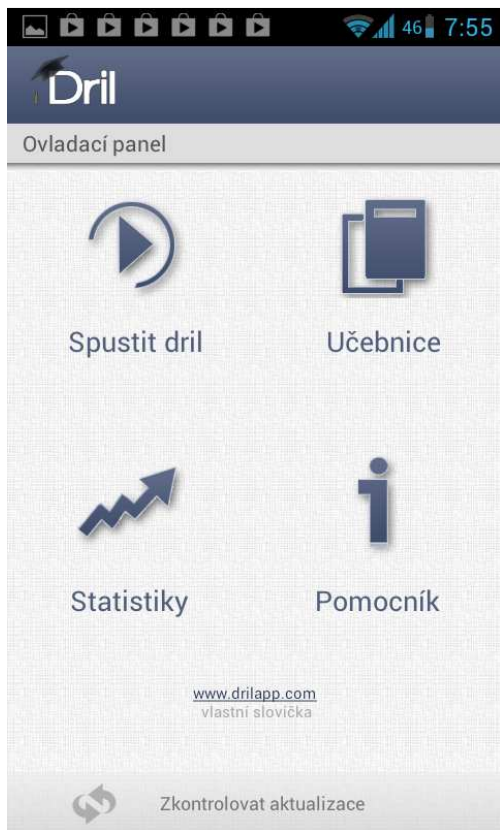
Obrázek 7: Dril - menu
