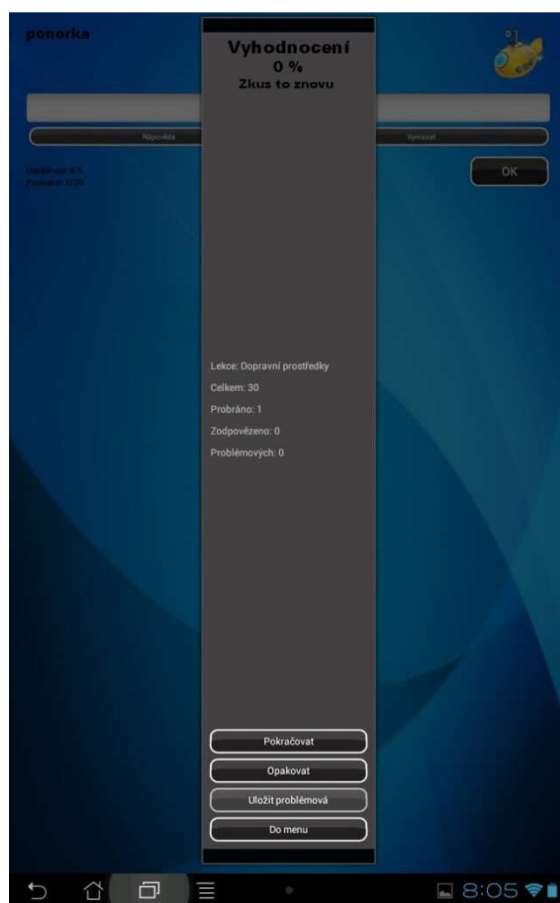
Obrázek 14: TrainBrain - roztažení
