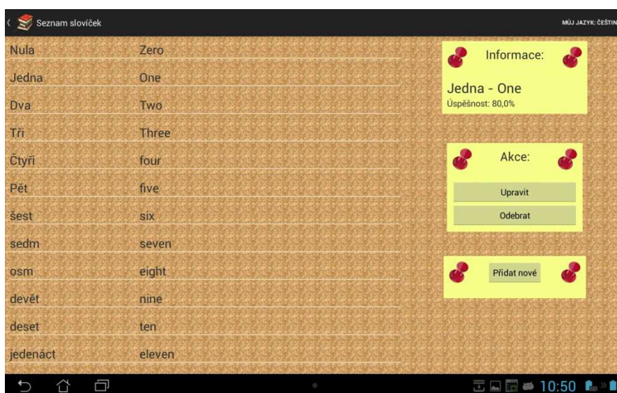
Obrázek 24: Seznam slovíček
