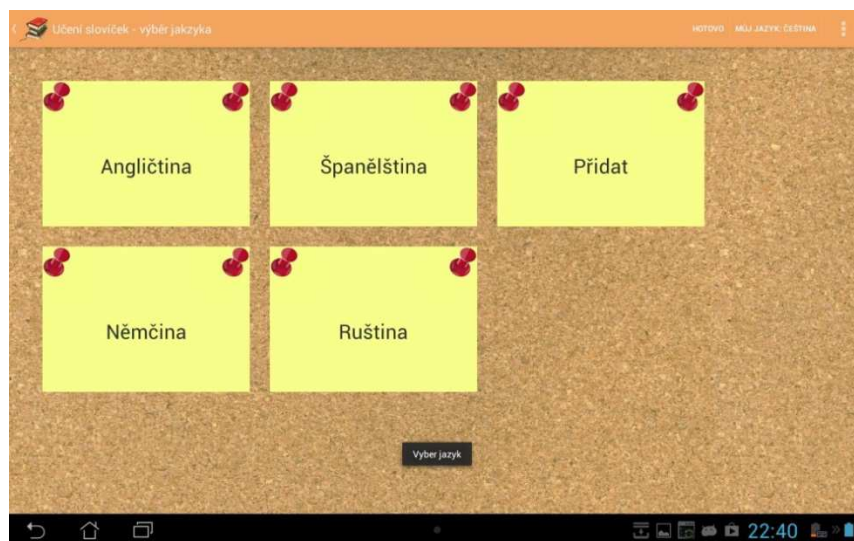
Obrázek 28: Toast
