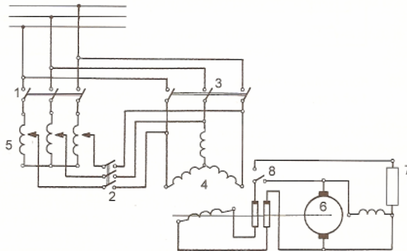
8 Schéma spouštění synch. motoru pomocí autotransf. (převzato z [11])
