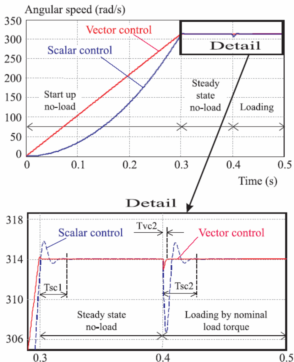
23 Dynamické srovnání skalárního / vektorové řízení PMSM (převzato [14])
