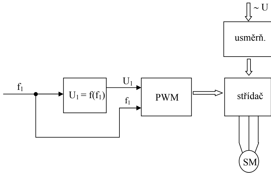
14 Frekvenčně napět'ové řízení s otevřenou smyčkou [8]
