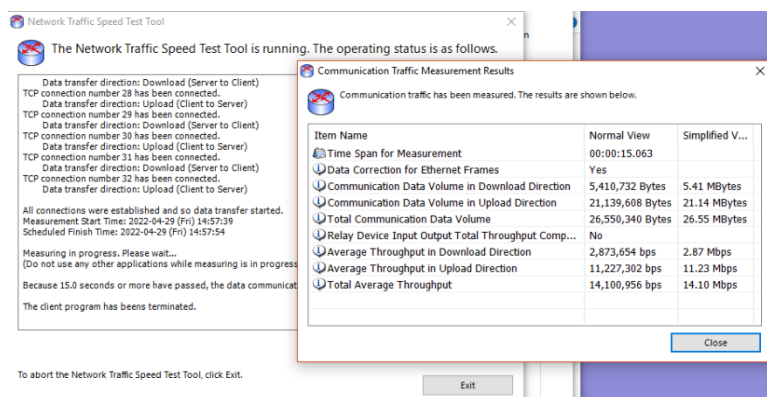
Obr. 37 Test rychlosti.
