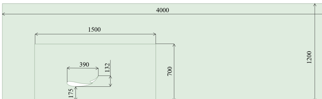
Obrázok 28: Rozmery optimalizovaného krídla a výpočtovej domény
