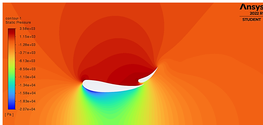
Obrázok 30: Kontúry statických tlakov okolo optimalizovaného krídla
