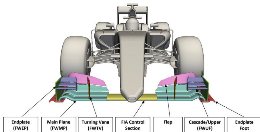
Obrázok 14: Jednotlivé aerodynamické prvky krídla, upravené z [23]
