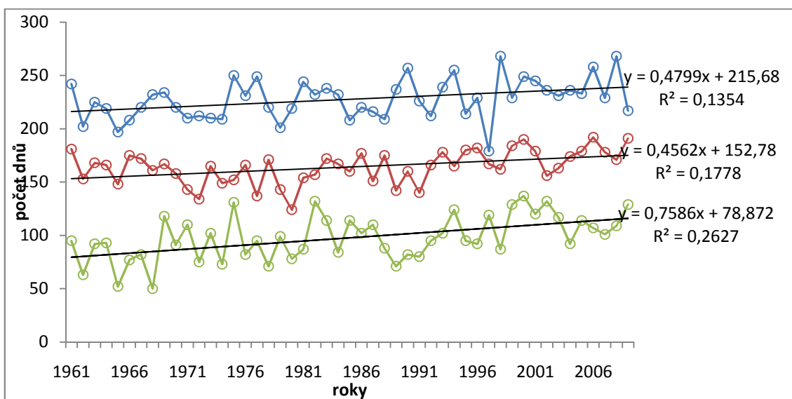
Obr. 8 Délka trvání ve dnech vegetačního léta (zelená), hlavního vegetačního období (červená), velkého vegetačního období (modrá) v průběhu let 1961 – 2009 na klimatologické stanici Velké Meziříčí.
