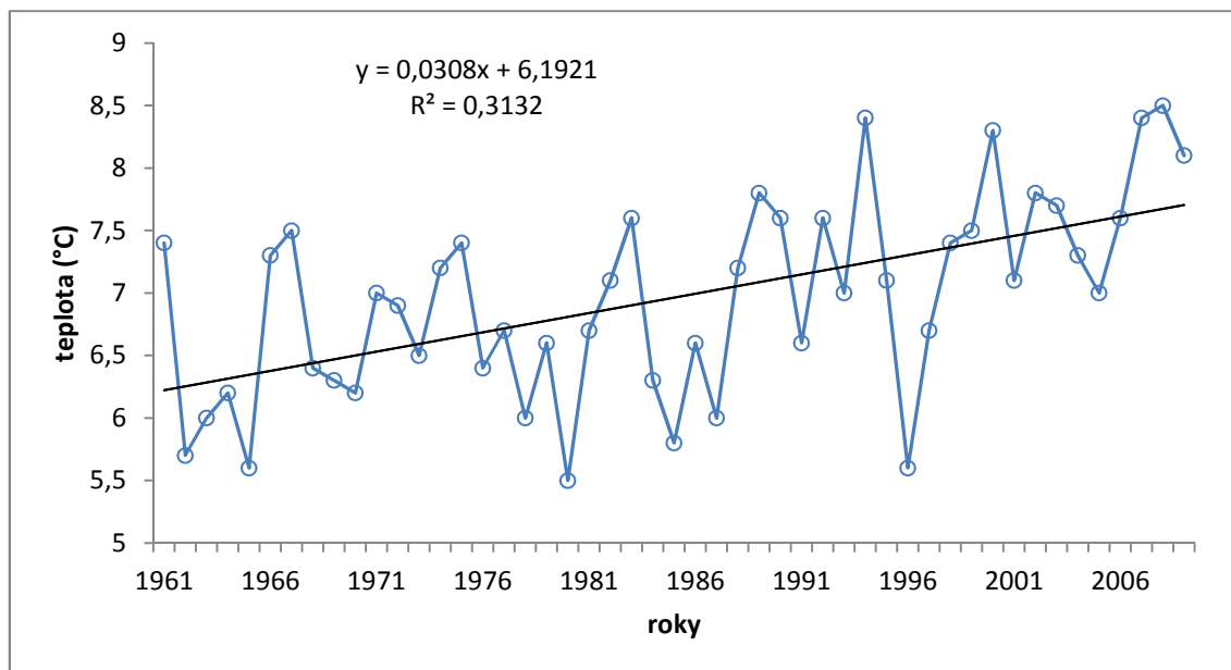
Obr. 11 Průměrná roční teplota vzduchu za období let 1961 – 2009 na klimatologické stanici Bystřice nad Pernštejnem.
