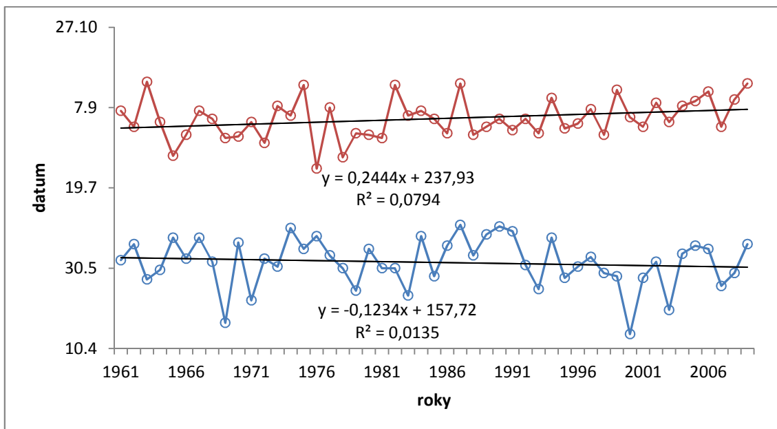
Obr. 14 Datum nástupu (modrá čára) a datum konce (červená čára) vegetačního léta období v průběhu let 1961 – 2009 na klimatologické stanici Bystřice nad Pernštejnem.
