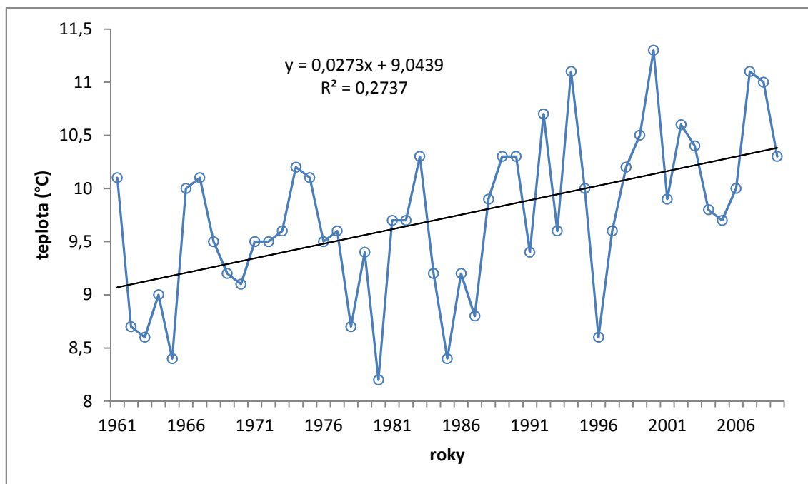
Obr. 17 Průměrná roční teplota vzduchu za období let 1961 – 2009 na klimatologické stanici Velké Pavlovice.
