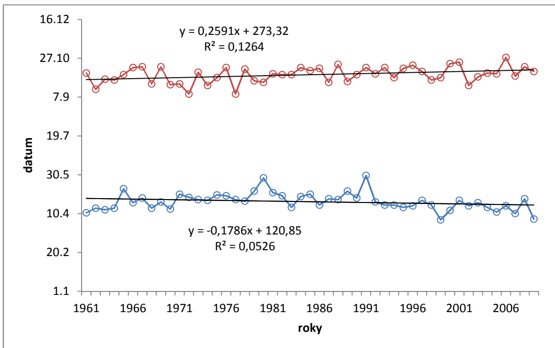
Obr. 6 Datum nástupu (modrá čára) a datum konce (červená čára) hlavního vegetačního období v průběhu let 1961 – 2009 na klimatologické stanici Velké Meziříčí.
