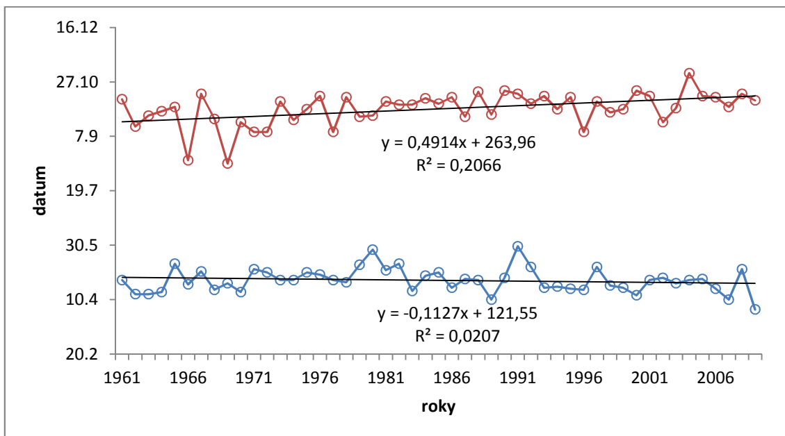
Obr. 13 Datum nástupu (modrá čára) a datum konce (červená čára) hlavního vegetačního období v průběhu let 1961 – 2009 na klimatologické stanici Bystřice nad Pernštejnem.
