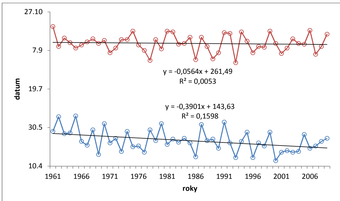
Obr. 20 Datum nástupu (modrá čára) a datum konce (červená čára) vegetačního léta v průběhu let 1961 – 2009 na klimatologické stanici Velké Pavlovice.
