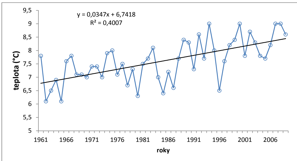
Obr. 4 Průměrná roční teplota vzduchu za období let 1961 – 2009 na klimatologické stanici Velké Meziříčí.
