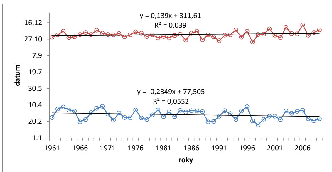
Obr. 18 Datum nástupu (modrá čára) a datum konce (červená čára) velkého vegetačního období v průběhu let 1961 – 2009 na klimatologické stanici Velké Pavlovice.
