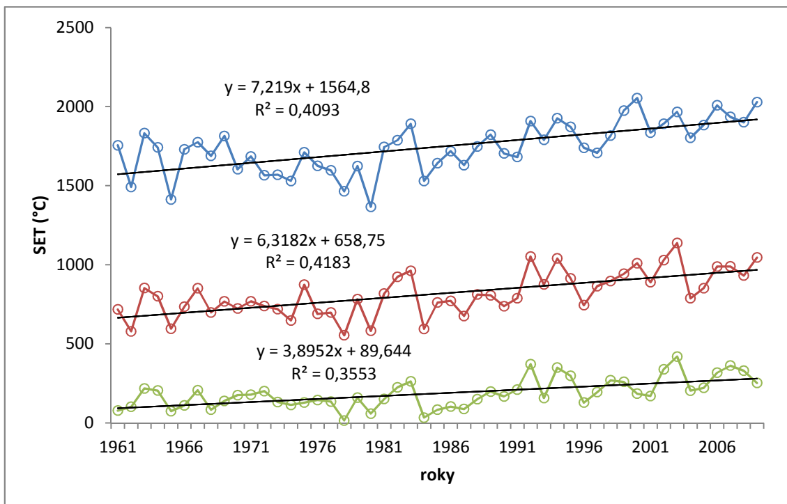
Obr. 9 Sumy efektivních teplot za vegetační léto (zelená), hlavní vegetační období (červená), velké vegetační období (modrá) v průběhu let 1961 – 2009 na klimatologické stanici Velké Meziříčí.
