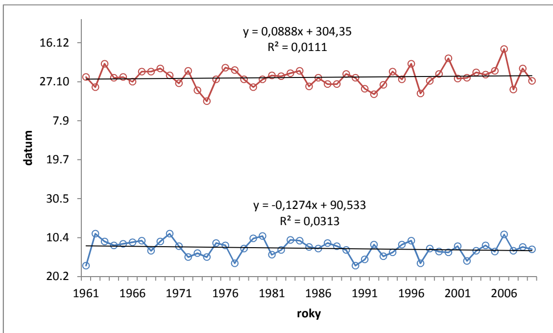
Obr. 12 Datum nástupu (modrá čára) a datum konce (červená čára) velkého vegetačního období v průběhu let 1961 – 2009 na klimatologické stanici Bystřice nad Pernštejnem.
