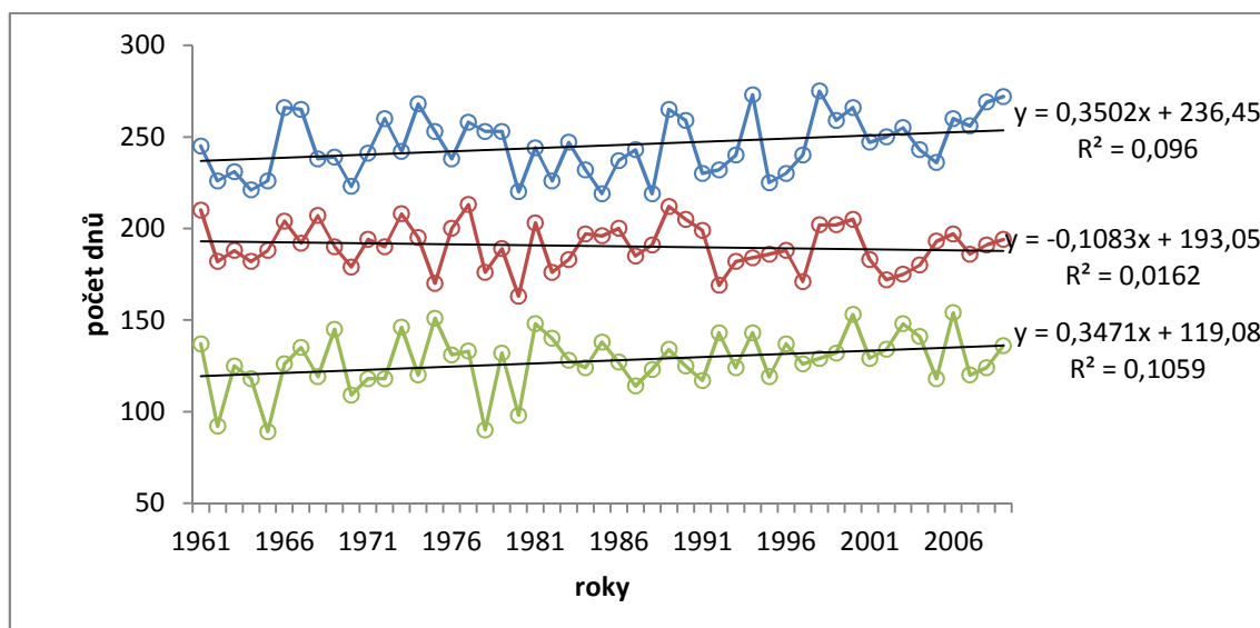
Obr. 21 Délka trvání ve dnech vegetačního léta (zelená), hlavního vegetačního období (červená), velkého vegetačního období (modrá) v průběhu let 1961 – 2009 na klimatologické stanici Velké Pavlovice.
