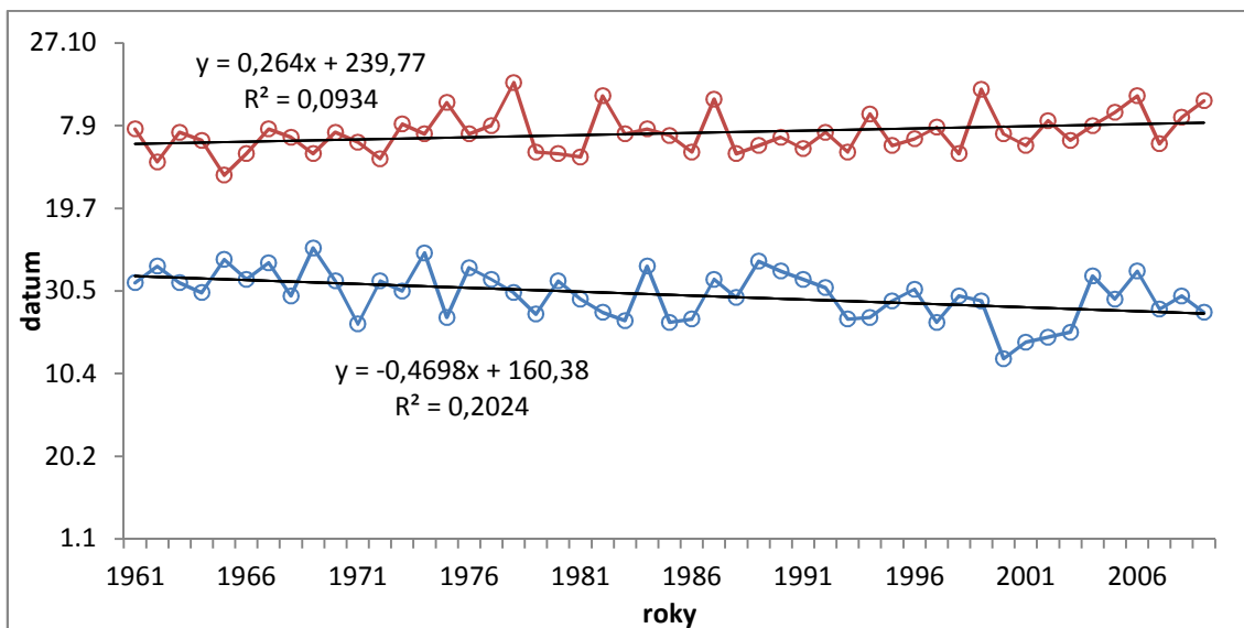
Obr. 7 Datum nástupu (modrá čára) a datum konce (červená čára) vegetačního léta v průběhu let 1961 – 2009 na klimatologické stanici Velké Meziříčí.
