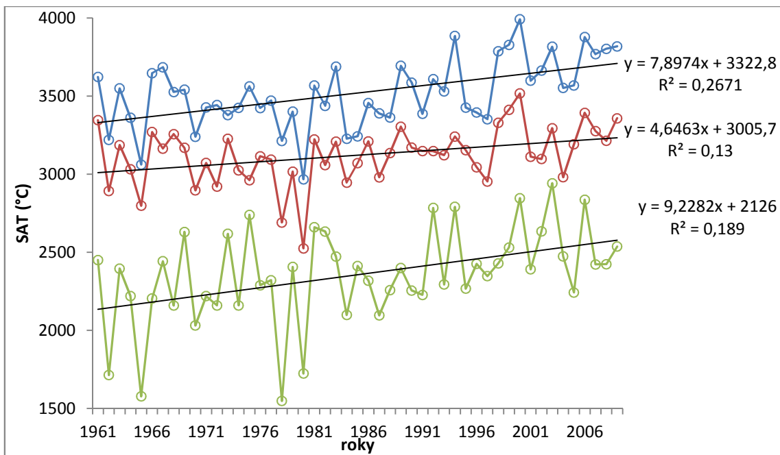
Obr. 23 Sumy aktivních teplot za vegetační léto (zelená), hlavní vegetační období (červená), velké vegetační období (modrá) v průběhu let 1961 – 2009 na klimatologické stanici Velké Pavlovice.
