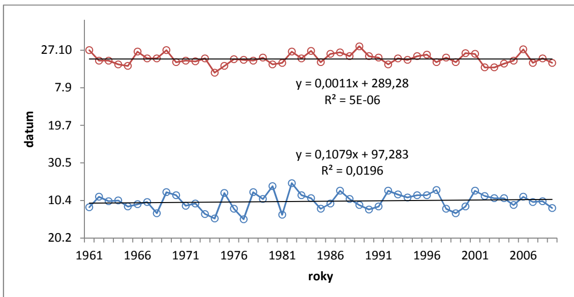
Obr. 19 Datum nástupu (modrá čára) a datum konce (červená čára) hlavního vegetačního období v průběhu let 1961 – 2009 na klimatologické stanici Velké Pavlovice.
