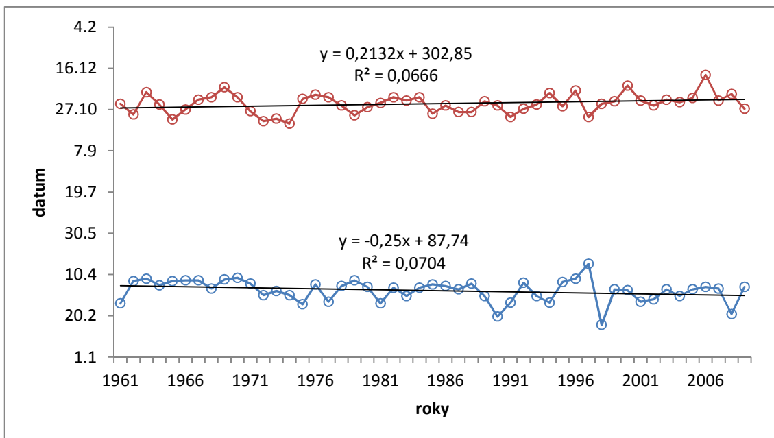
Obr. 5 Datum nástupu (modrá čára) a datum konce (červená čára) velkého vegetačního období v průběhu let 1961 – 2009 na klimatologické stanici Velké Meziříčí.
