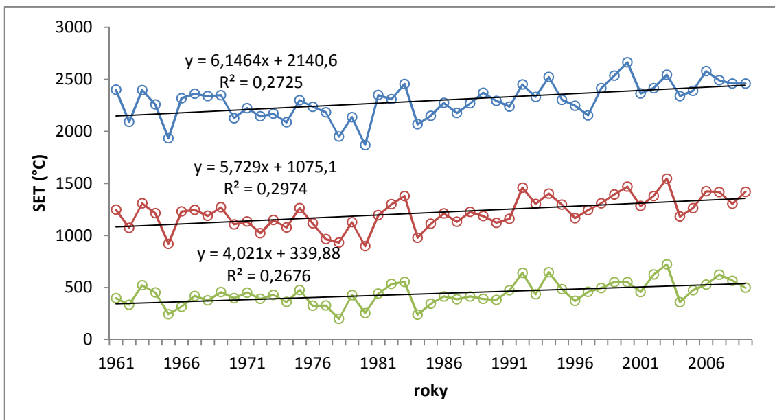
Obr. 22 Sumy efektivních teplot za vegetační léto (zelená), hlavní vegetační období (červená), velké vegetační období (modrá) v průběhu let 1961 – 2009 na klimatologické stanici Velké Pavlovice.
