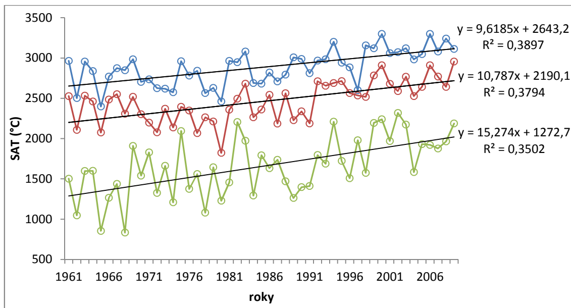
Obr. 10 Sumy aktivních teplot za vegetační léto (zelená), hlavní vegetační období (červená), velké vegetační období (modrá) v průběhu let 1961 – 2009 na klimatologické stanici Velké Meziříčí.
