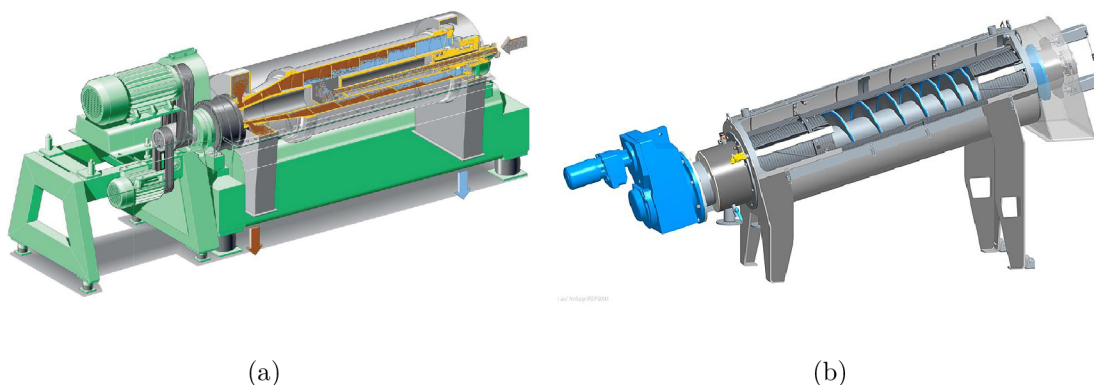
Obr. 2.13: (a) Dekantační odstředivka [44], (b) Šnekový lis[43]
