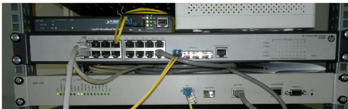
Obr. 4.3: Zapojení části testovacího polygonu ve stojanu.
