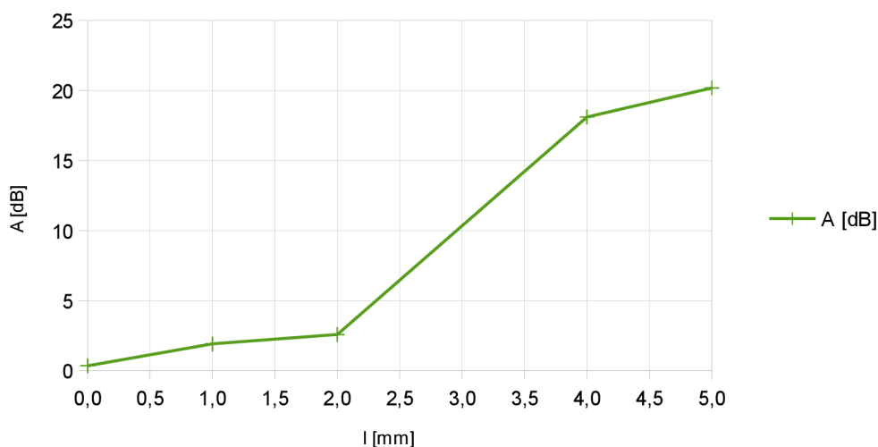
Obr. 4.9: Graf závislosti útlumu optického výkonu na příčné odchylce.
