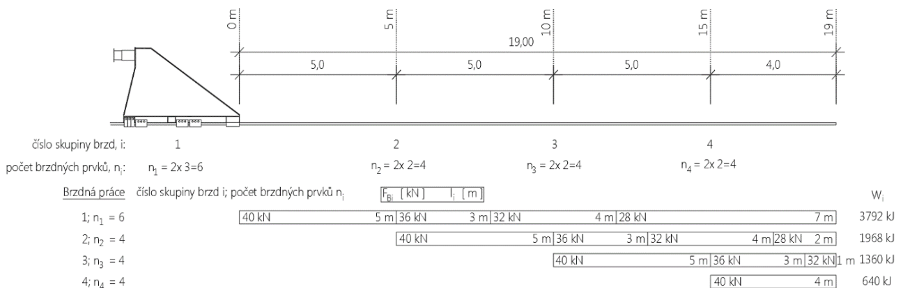
Obr. 6.3 Rozdělení brzdě dráhy do dílčích úseků
