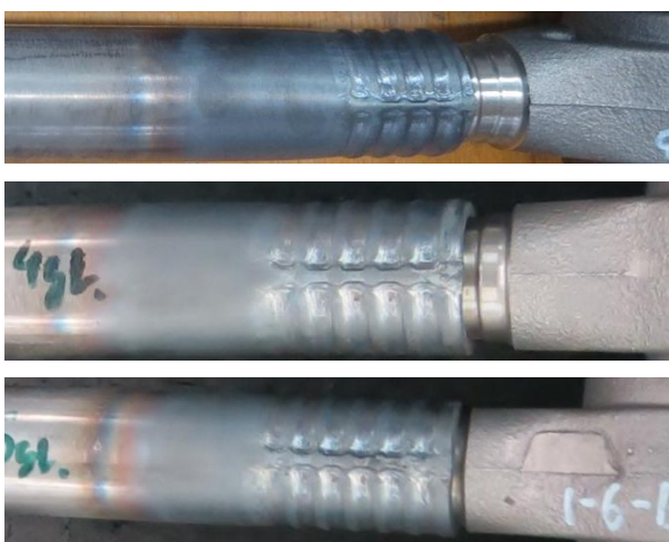
Obr. 34 Spoj trubka \text{\O} 48 \times 5 mm spolu s 3,4,5 drážkami
