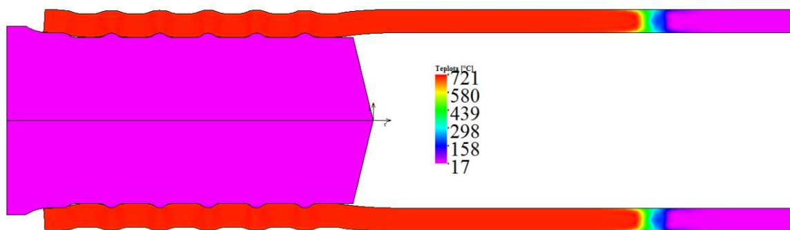
Obr. 23 Teplotní pole (100% výpočtu )
