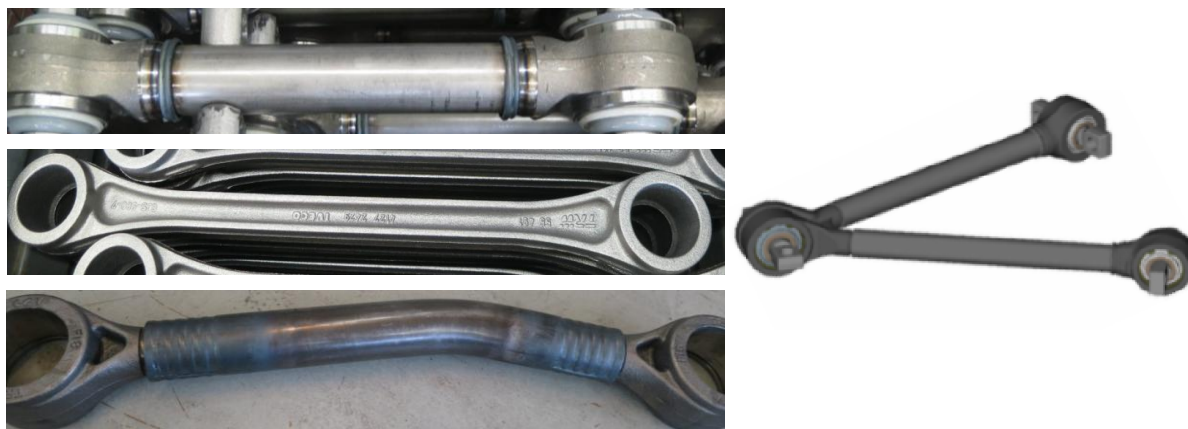
Obr. 6 Příklad táhel vyrobených různými technologiemi [10]
