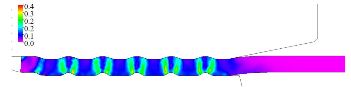
Obr. 27 Log. přetvoření (100% výpočtu)
