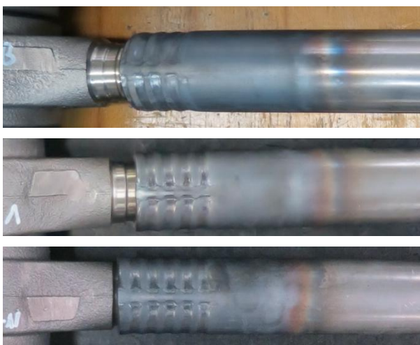
Obr. 35 Spoj trubka \text{\O} 50 \times 6 mm spolu s 3,4,5 drážkami
