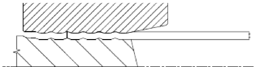
Obr. 31 výroba prototypů-varianta 2
