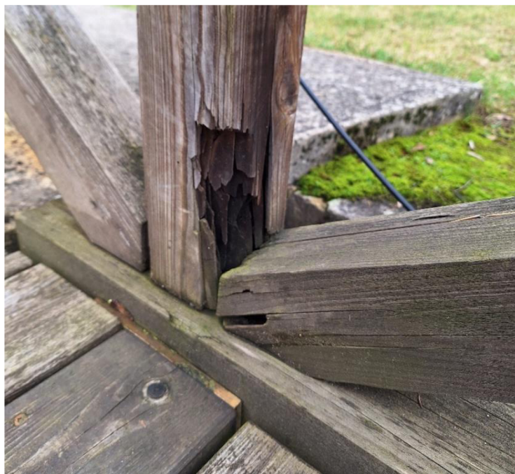
Obrázek 35-Poškození spoje sloupků a vzpěr nosníku (autor)
