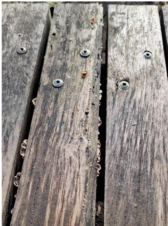
Obrázek 24-Poškození trámu vedlejšího pole mostu (autor)
