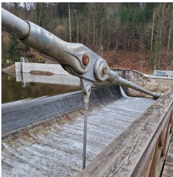
Obrázek 31-Připojení závěsů ve spoji táhel (autor)
