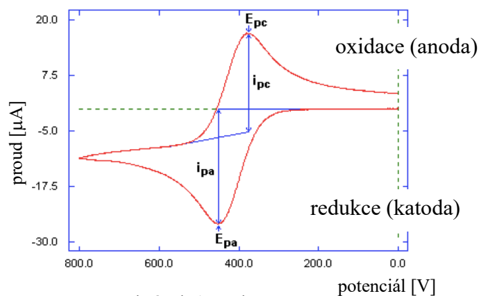
Obrázek 1: Voltamogram
