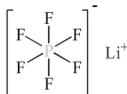
Obrázek 9: Struktura soli LiPF 6 [4]
